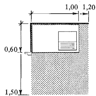
Figur 63:21 g. Tvättbänk (1,00 × 0,60 m och 1,20 × 0,60 m).
