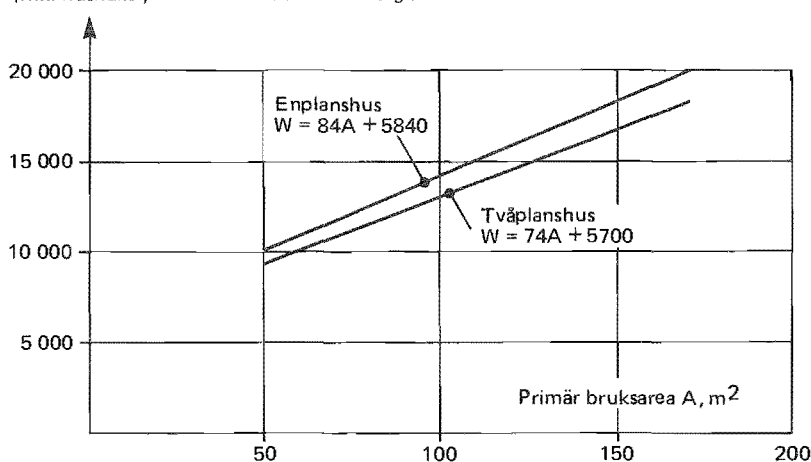
Figur 39:931. Godtaget årsenergibehov som funktion av primär bruksarea i direktelvärmda energisnåla småhus
