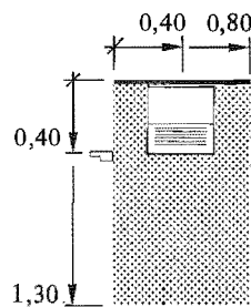
Figur 63:21 f. Tvättlåda (0,40 × 0,40 m).
