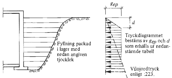
Figur 22:251. Jordtryck vid packad återfyllning av friktionsjord.
