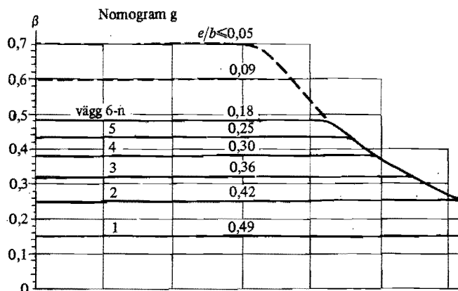
Figur 24:422 f-g. Godtagna reduktionsfaktorer för väggar med från båda sidor anslutande bjälklag (innerväggar) eller då e/b är känt. Nomogram f gäller vid enkelspända bjälklag i byggnader med två fack när l_1/l_2 \leq 0,8 och l_2 \leq 5,0 m. Nomogram g gäller vid enkelspända bjälklag i byggnader med tre eller flera fack med spännvidden högst 5 m samt där e bestäms enligt figuren.
