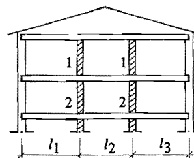
Figur 24:422 f-g. Godtagna reduktionsfaktorer för väggar med från båda sidor anslutande bjälklag (innerväggar) eller då e/b är känt. Nomogram f gäller vid enkelspända bjälklag i byggnader med två fack när l_1/l_2 \leq 0,8 och l_2 \leq 5,0 m. Nomogram g gäller vid enkelspända bjälklag i byggnader med tre eller flera fack med spännvidden högst 5 m samt där e bestäms enligt figuren.
