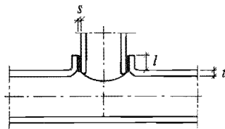
Avgrening med utkrågning. Röret i kragen godtas inte hindra vattenströmningen i huvudröret.
