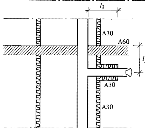
Figur 52:331 a. Godtaget utförande av en oisolerad kanal i ett stängt schakt. Beteckningar enligt figur 52:33 a. Villkor enligt figurerna 52:33 b-c.
