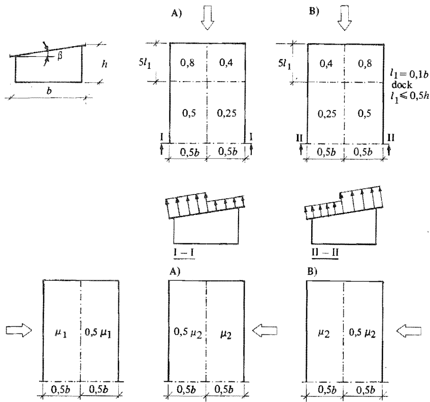
Figur 22:5332 b. Godtagna värden på formfaktorer för utväändig vindlast på pulpettak. A och B betecknar två olika lastfall, vilka båda förutsätts bli beaktade. \mu_1 och \mu_2 bestäms enligt diagram i figur 22:5332 a.
