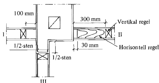
Figur 44:324 a. Godtagna vägganslutningar till en röckanal med enkel kanalvägg av tegelmurverk. Vid alternativ I (vägg med vertikala reglar) förutsätts regeln befinna sig minst 100 mm från röckkanalens vägg. Vid alternativ II (vägg med horisontella reglar) förutsätts ändytorna på reglarna befinna sig minst 30 mm från väggen och förekommande vertikala reglar minst 300 mm från väggen. Vid alternativ III godtas att såväl en vägghpanel som en träregel ansluts direkt mot en murklack.
