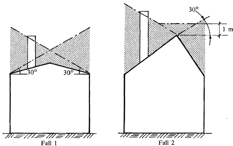
Figur 44:1222. Godtagen beräkning av höjd för rökanal till anläggning avsedd för tunnlolja, med tillförd värmeeffekt 0,06 < P \leq 50 MW. Principskiss. Av figurens nivålinjer framgår lägsta godtagbara höjd.
