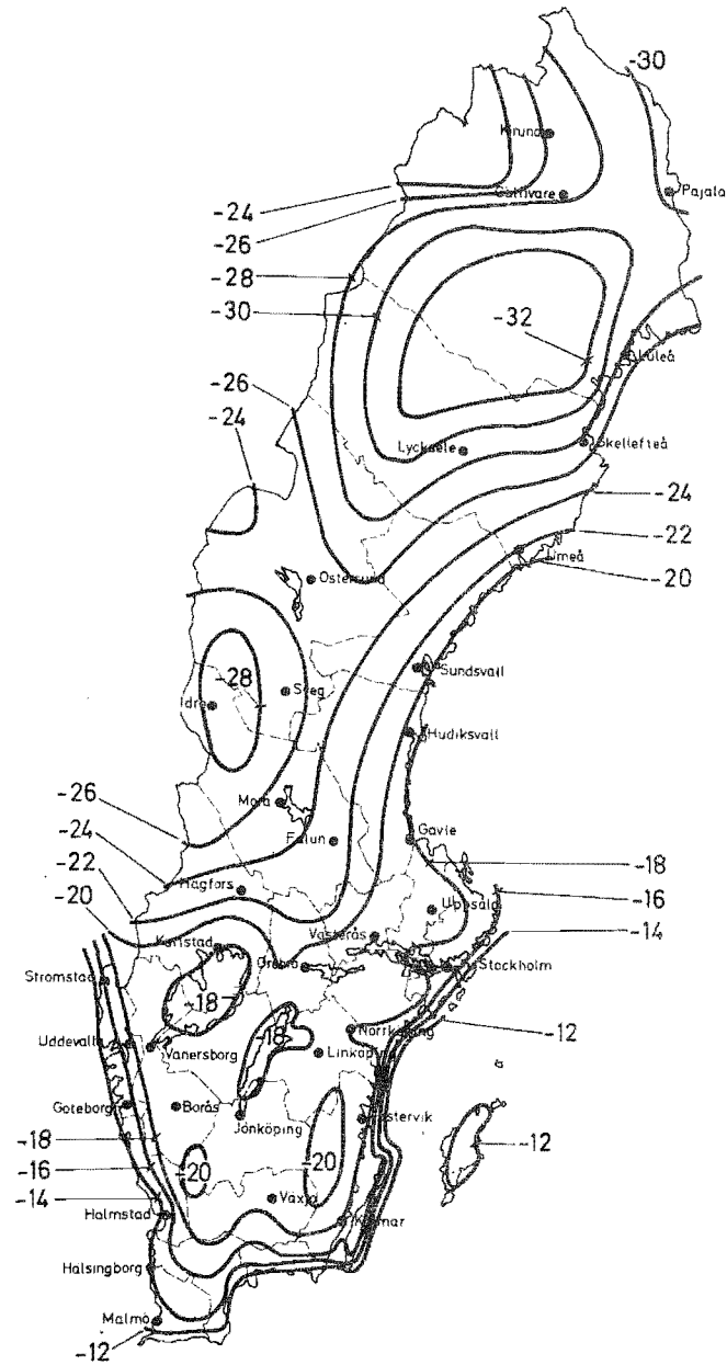
Figur 22:721. Godtagna dygnsmedelvärden för låga temperaturer.
