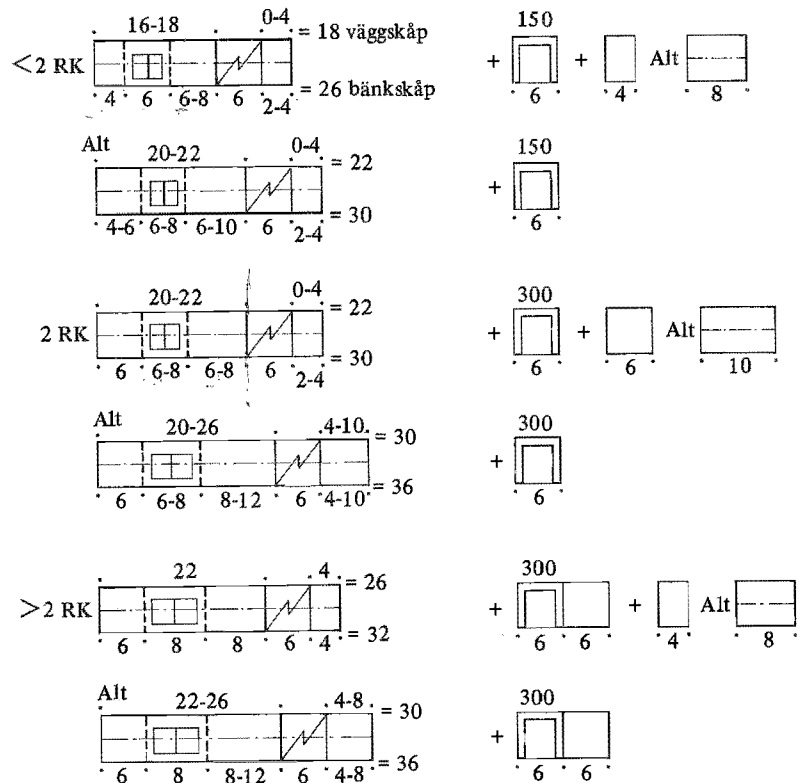
Figur 71:214. Delmått på godtagen minsta inrednings- och utrustningsmängd för olika lägenhetsstorlekar. Delmått anges i dm. 150 och 300 anger kylid volym i liter.
