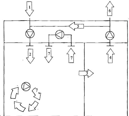
Figur 36:11 b. Benämningar på luftflöden.
