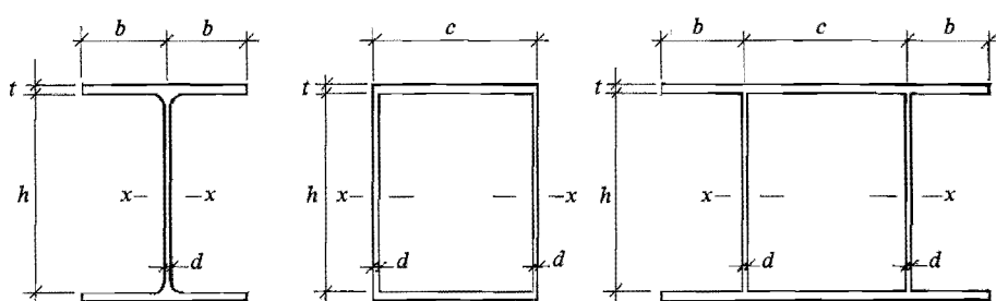
Figur 28:21. Beteckningar för tvärsnittsmått.
