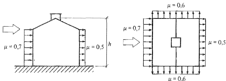
Figur 22:5331 a. Godtagna värden på formfaktorer för utvändigt vindlast på ytterväggar. Höjden h används för att bestämma det exceptionella hastighetstrycket enligt figur 22:52.
