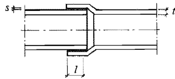
Rak överlappsfog.
