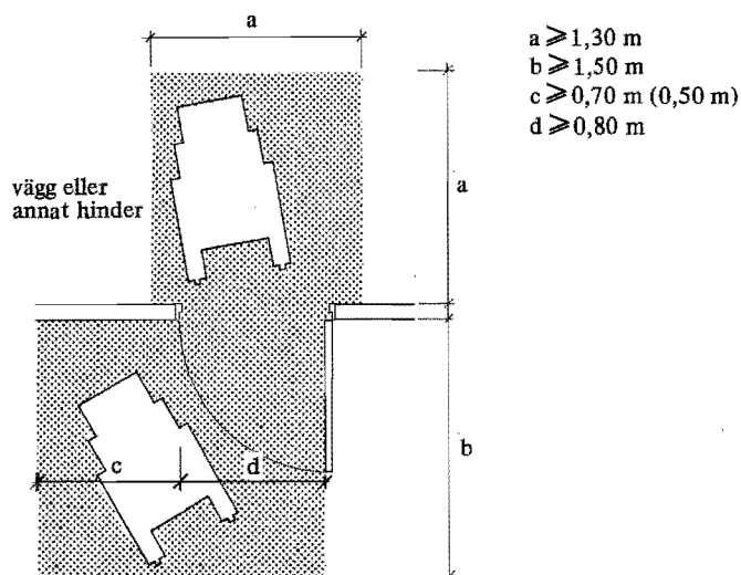
Figur 62:12. Entré för passage med rullstol.
