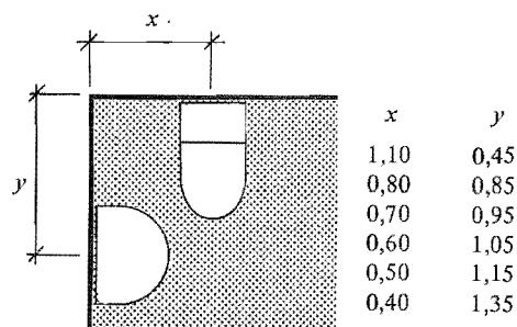
Figur 63:22. Exempel på godtagna kombinationsmått vid vinkeluppställning.
