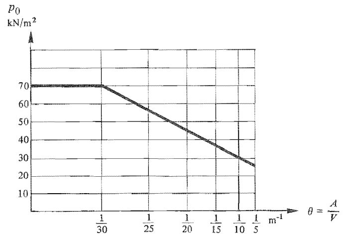
Figur 22:84. Antagna invändiga övertryck i en enda sluten lokal som funktion av faktorn \theta
