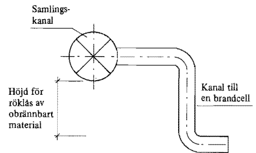
Figur 52:342. Godtagen princip för anordnande av röklås.
