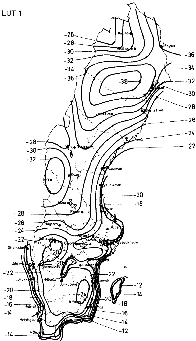
Figur 35:23 a. Isotermkarta som visar den dimensionerande lägsta utetemperaturer för hus av trä eller annan lätt byggnad, LUT 1. LUT-värden enligt figuren korrigeras om ifrågavarande byggnad ligger på en plats som bedöms vara kallare eller varmare än trakten i genomsnitt.
