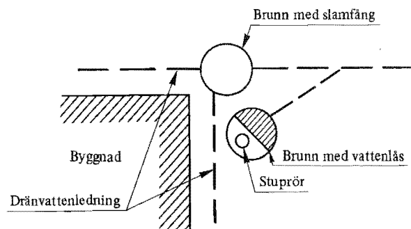
Figur 51:31 a. Exempel på godtaget sätt att ansluta dränvattenledning till dagvattenledning. Större installation.
