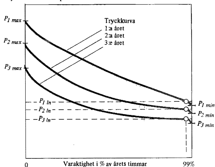
Figur 51:13. Definition av lägsta normala vattentryck.
