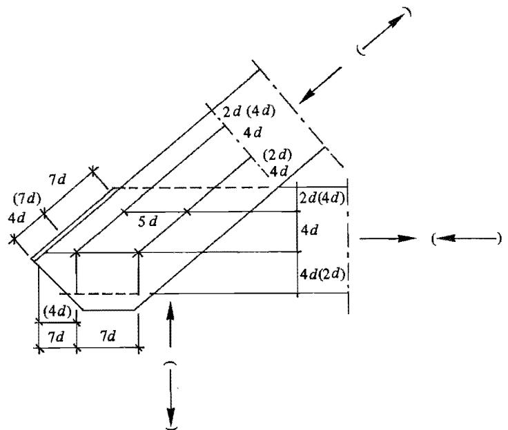
Figur 27:54. Förutsatta minimiavstånd mellan skruvar och från skruv till virkeskant i skruvförband utan mellanläggsbrickor. Värden inom parentes gäller för inom parentes angiven kraftpåverkan. ( d är skruvdiameter.)
