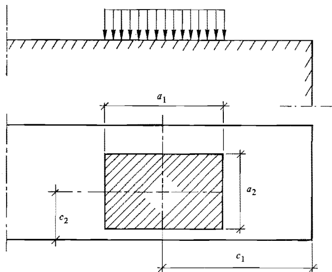
Figur 24:312. Beteckningar vid bestämning av lokalt tryck.
