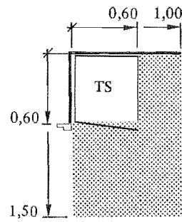
Figur 63:21 i. Torfskåp (0,60 × 0,60 m).
