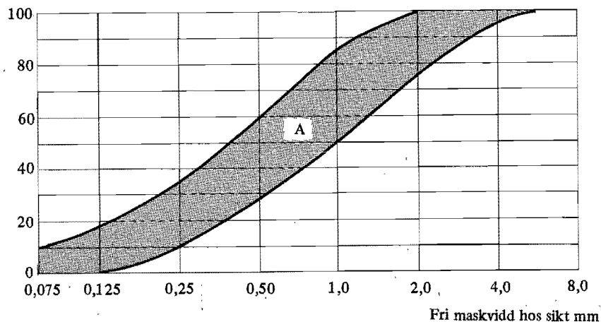
Figur 24:52. Godtagen kornfördelning för sand till murbruk vid normal fogtjocklek.
