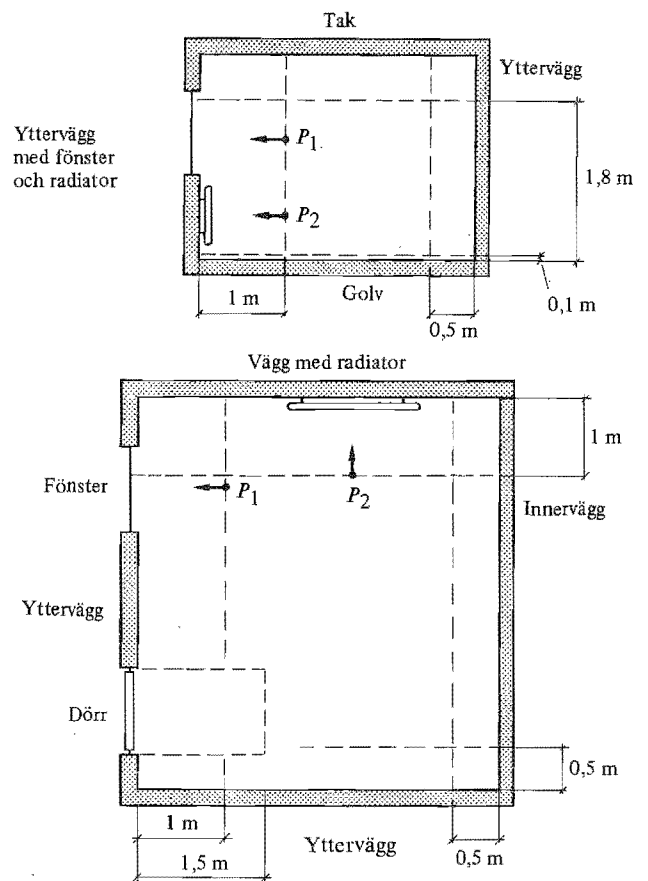
Figur 35:21. Exempel som visar kontrollzonens storlek och placering av punkterna P_1 och P_2 enligt 35:21.
