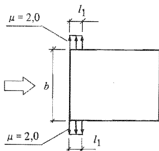
Figur 22:5331 a. Godtagna värden på formfaktorer för utvändigt vindlast på ytterväggar. Höjden h används för att bestämma det exceptionella hastighetstrycket enligt figur 22:52.
