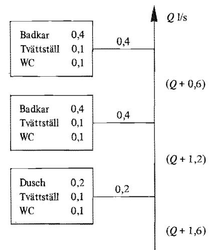
Figur 51:154. Godtagen beräkning av summerade normflöden vid dimensionering av fördelningsledning till badrum o d, l/s.
