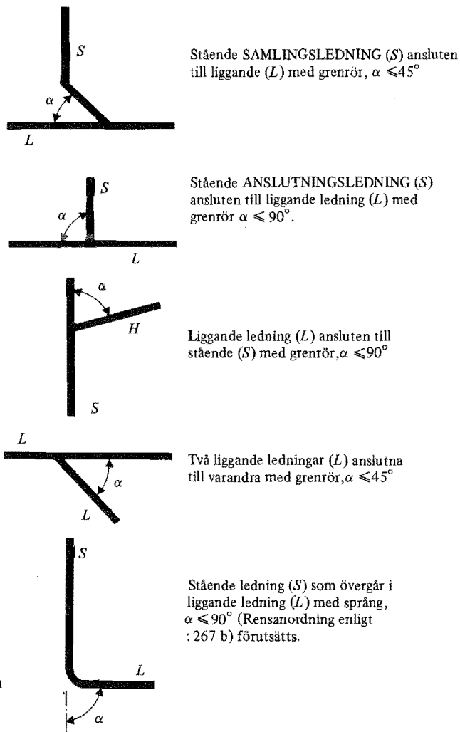
Figur 51:2632. Godtagna största vinkelmått mellan spillvattenledningar i byggnad.
