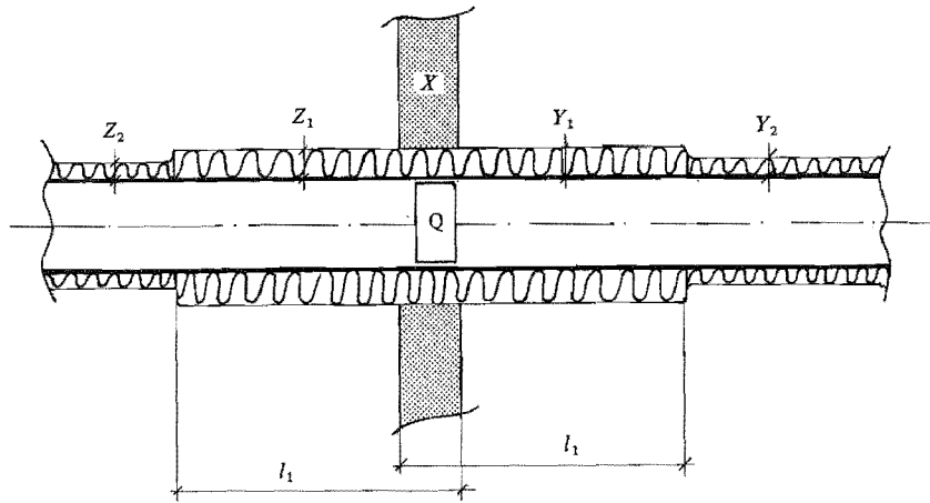
Figur 52:33 b. Godtagen brandteknisk klass hos en kanalvägg vid genombrott av en brandcellsskiljande byggnadsdel. Beteckningar enligt figur 52:33 a.
