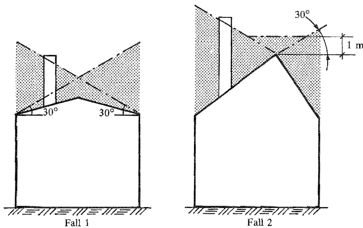
Figur 44:1222. Godtagen beräkning av höjd för rökkanal till anläggning avsedd för tunnlja, med tillförd värmeeffekt 0,06 < P \leq 50 MW. Principskiss. Av figurens nivålinjer framgår lägsta godtagbara höjd.
