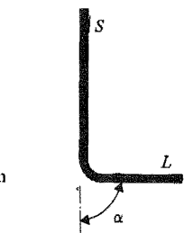
Figur 51:2632. Godtagna största vinkelmått mellan spillvattenledningar i byggnad.
