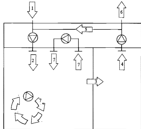
Figur 36:11 b. Benämningar på luftflöden.
