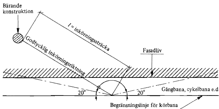
Figur 22:82 b. Antagna inkörningsriktningar och inkörningssträckor.
