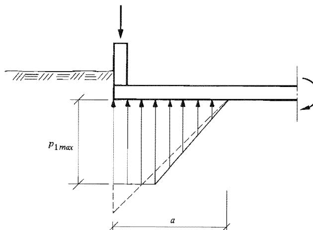
Figur 23:262 b. Omfördelning av den triangulära tryckfördelningen när det beräknade grundtrycket vid plattans kant p_1 överskrider p_{1max} .
