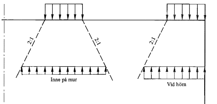
Figur 24:41 a. Godtagen tryckutbredning under ett upplag.
