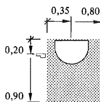
Figur 63:21 b. Handtvättställ (0,50 × 0,35 m).
