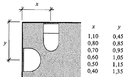
Figur 63:22. Exempel på godtagna kombinationsmått vid vinkeluppställning.
