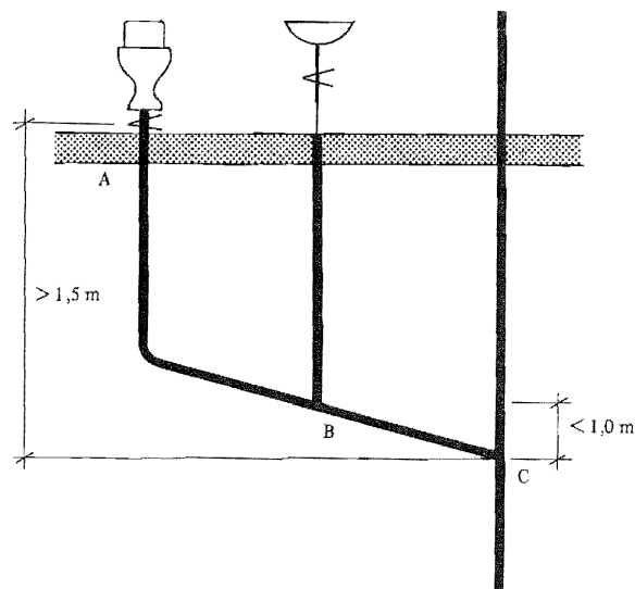
Figur 51:2431. Begränsningar för anslutning av avloppsenhet till oluftad anslutningsledning från en vattenklosett.
