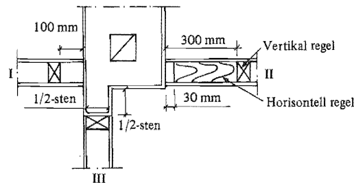
Figur 44:324 a. Godtagna vägganslutningar till en rökkanal med enkel kanalvägg av tegelmurverk. Vid alternativ I (vägg med vertikala reglar) förutsätts regeln befinna sig minst 100 mm från rökkanalens vägg. Vid alternativ II (vägg med horisontella reglar) förutsätts ändytorna på reglarna befinna sig minst 30 mm från väggen och förekommande vertikala reglar minst 300 mm från väggen. Vid alternativ III godtas att såväl en väggsplatt som en träregel ansluts direkt mot en murklack.
