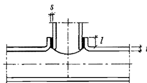
Avgrening med utkragning. Röret i kragen godtas inte hindra vattenströmningen i huvudröret.
