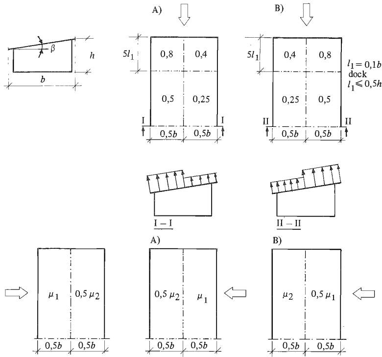
Figur 22:5332 b. Godtagna värden på formfaktorer för utväändig vindlast på pulpet-tak. A och B betecknar två olika lastfall, vilka båda förutsätts bli beaktade. \mu_1 och \mu_2 bestäms enligt diagram i figur 22:5332 a.
