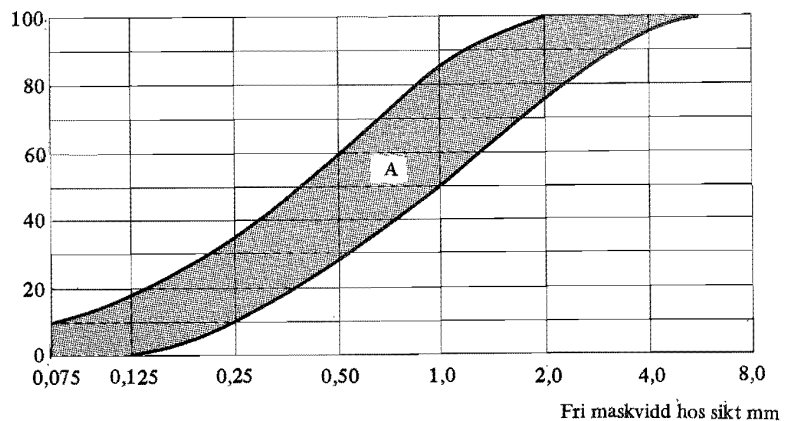
Figur 24:52. Godtagen kornfördelning för sand till murbruk vid normal fogtjocklek.
