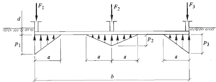
Figur 23:262 a. Grundtryckets fördelning under hel bottenplatta.
