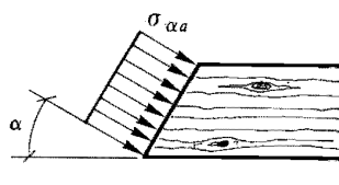
Figur 21:212 b. Tryckpåkänning i sned vinkel mot fiberriktningen.
