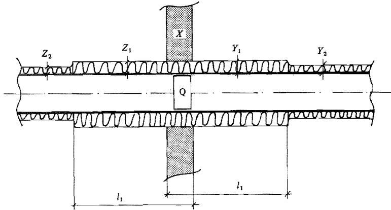
Figur 52:33 b. Godtagen brandteknisk klass hos en kanalvägg vid genombrott av en brandcellsskiljande bygnadsdel. Beteckningar enligt figur 52:33 a.
