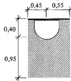
Figur 63:23 a. Tvättställ (vattenlås och avloppsrör placerat åt sidan eller i vägg).
