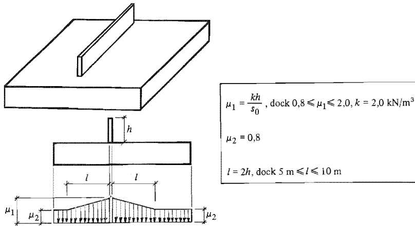
Figur 22:43 c. Godtagna formfaktorer för snölast vid skärm. Beträffande förutsättningar se faktaruta ovan.
