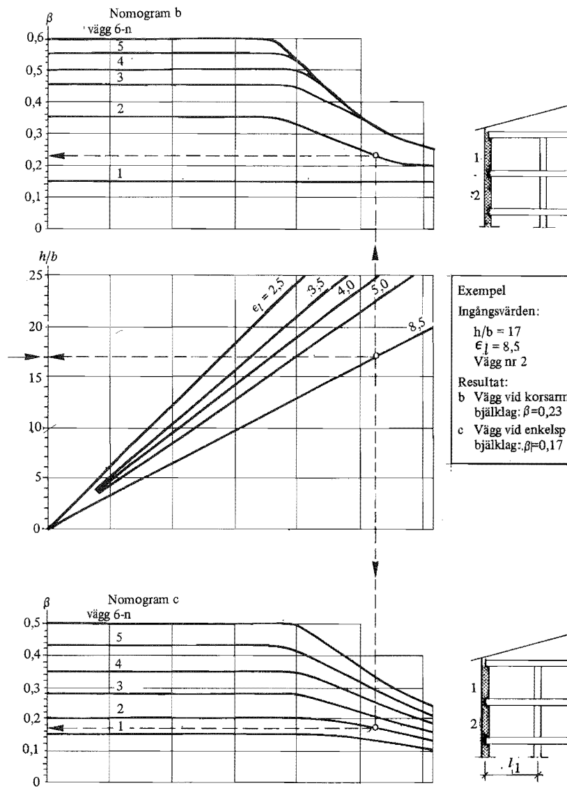
Figur 24:422 b-c. Godtagna reduktionsfaktorer för väggar med från en sida anslutande bjälklag (ytterväggar och liknande). Nomogram b gäller vid korsarmerade bjälklag med minsta spännvidden max 5,0 m. Nomogram c gäller vid enkelspända bjälklag l_1 \leq 5,0 m.
