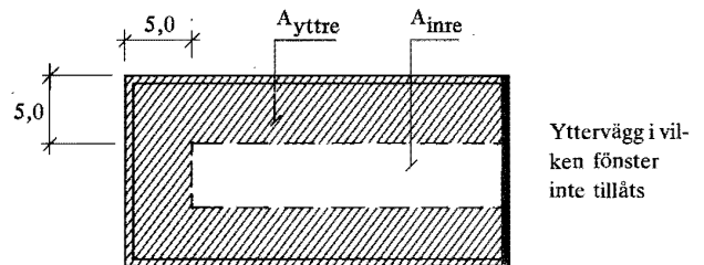
Figur 33:212. Exempel på beräkning av tillåten fönsterarea. Om husets längd är 40 m och dess bredd 15 m blir fönsterarean: 0,15 (40 \cdot 10 + 5 \cdot 5) + 0,03 \cdot 5 \cdot 35 = 69 \text{ m}^2 per våningsplan.
