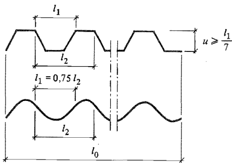
Figur 22:535 a. Godtagen bestämning av vindlastens komponent parallellt med en yta med tvärställda ribbor eller korrugeringar. Beteckningar för beräkning av formfaktorn för tangentiell vindlast.
