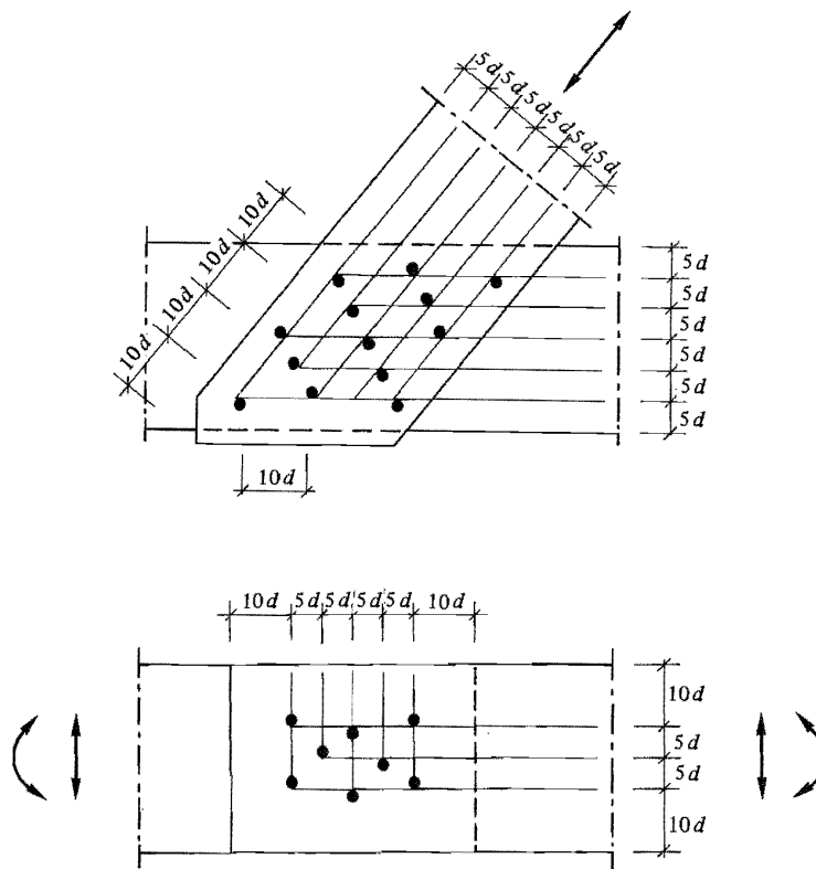
Figur 27:52 a. Förutsatt minimiavstånd mellan spikar och från spik till kant för virke och K-skivor och till virkesände ( d är spikens tvärrmått). Där två avstånd anges gäller det större.
