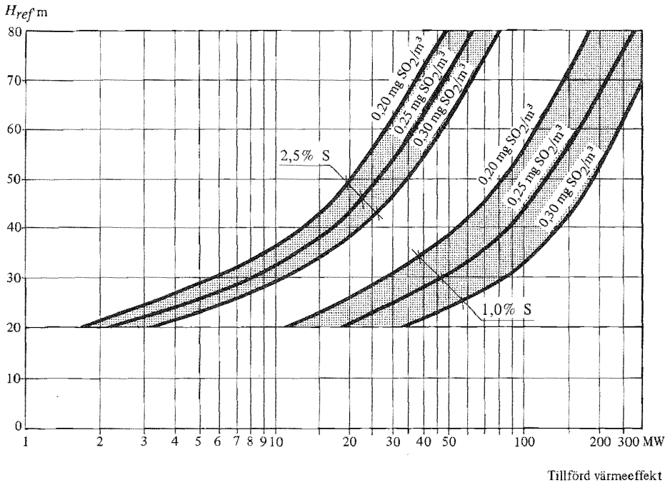
Figur 44:1223 a. Godtagen beräkning av rökkanalers referenshöjd H_{ref} vid anläggning för tjockolja. H_{ref} förutsätts inte underskrida 20 m.
