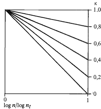
Figur 21:5213 b. Typiserade lastkollektiv.
