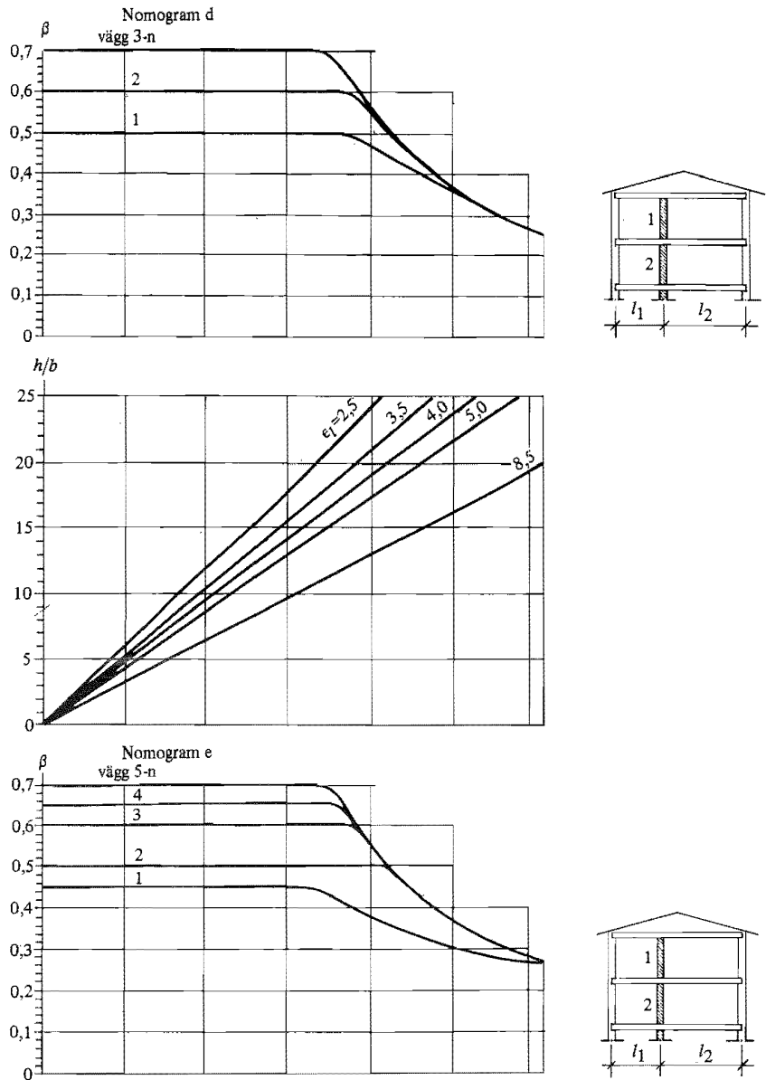
Figur 24:422 d-e. Godtagna reduktionsfaktorer för väggar med från båda sidor anslutande bjälklag (innerväggar).
