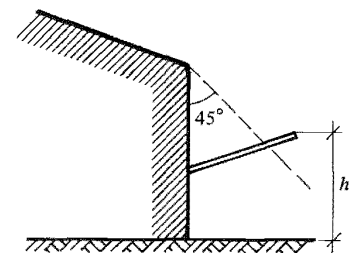
Figur 22:5344 b. Skärmtak i direkt anslutning till vägg med en del av skärmtaket utanför en 45^\circ -linje från byggnadens takfot. Beträffande vindbelastning se :5332.
