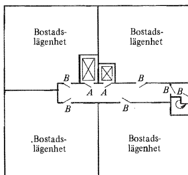
Figur 37:127. Principskiss med exempel på våningsplan vid brand- och röksäkert trapphus i bostadshus. Beteckningar enligt figur 37:126.
