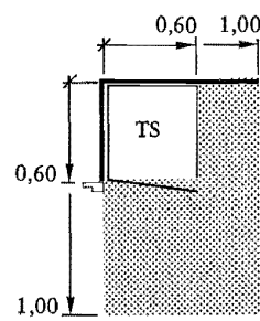
Figur 63:21 i. Torkskåp (0,60 × 0,60 m).
