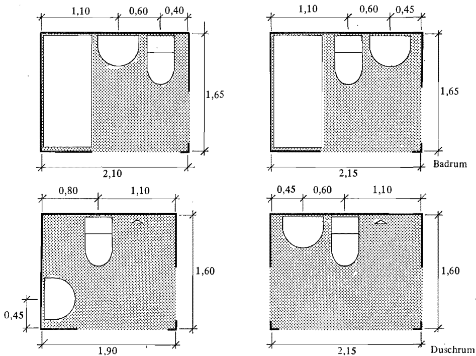
Figur 63:23 e. Hygienrum i bostäder som kan användas för toalettbesök av person med god rörlighet i rullstol. Efter ändring av inredningen kan rummen också användas av dessa för personlig hygien.
