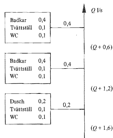
Figur 51:154. Godtagen beräkning av summerade normflöden vid dimensionering av fördelningsledning till badrum o d, l/s.
