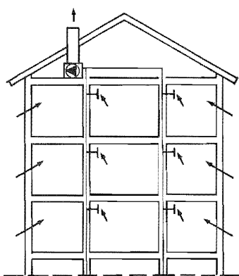
Typ F Ventilation med fläktstyrda frånluftsflöden
