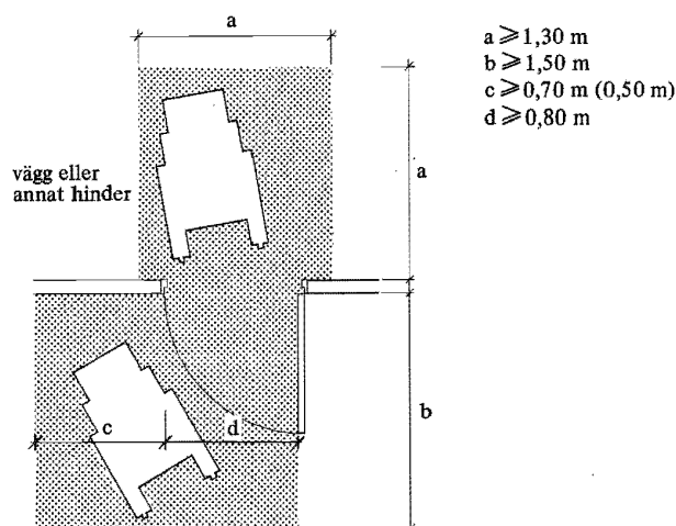
Figur 62:12. Entré för passage med rullstol.
