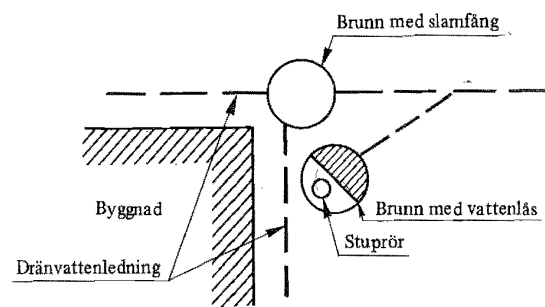
Figur 51:31 a. Exempel på godtaget sätt att ansluta dränvattenledning till dagvattenledning. Större installation.
