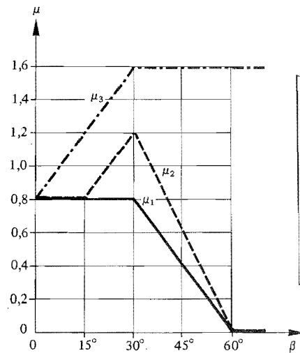
Figur 22:43 a. Godtagna formfaktorer för snölast på sadeltak och i fråga om snölastens effekter jämförbara tak. Beträffande förutsättningar se faktaruta ovan.
