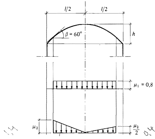
Figur 22:43 b. Godtagna formfaktorer för snölast på bågtag. Beträffande alternativa lastfall se faktaruta ovan.
