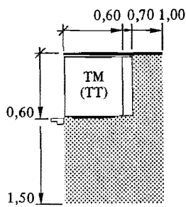
Figur 63:21 h. Tvättmaskin, torktumlare (0,60 × 0,60 m).
