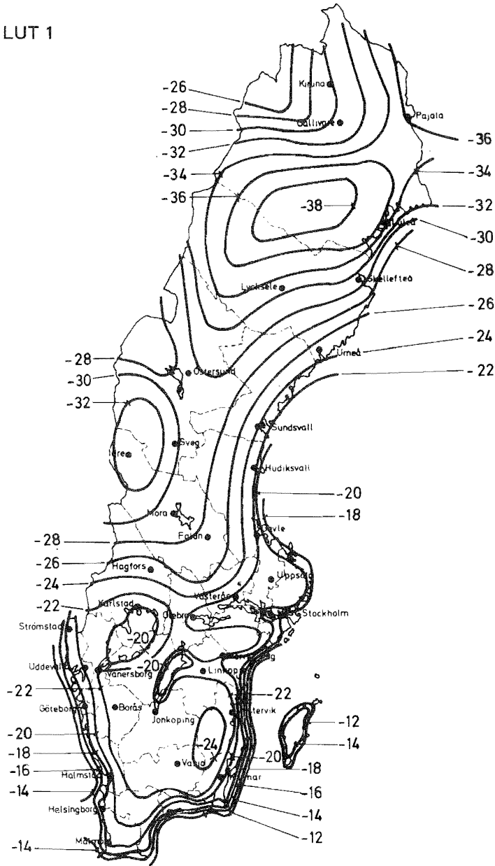
Figur 35:23 a. Isotermkarta som visar den dimensionerande lägsta utetemperaturen för hus av trä eller annan lätt byggnad, LUT 1. LUT-värden enligt figuren korrigeras om ifrågasvarande byggnad ligger på en plats som bedöms vara kallare eller varmare än trakten i genomsnitt.
