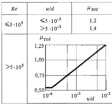
Figur 22:5341 b. Godtagna värden på formfaktorer för cylindriska stänger med l > 5d . Re är Reynolds tal och u är höjden på ojämnheter på stångytan.
