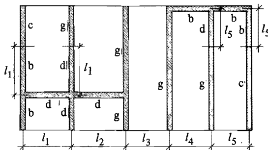
Figur 24:422 a. Väggpartierna b, c, d och g, för vilka nomogrammen i figurerna 24:422 b–g gäller.
