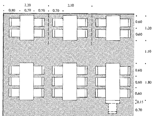
Figur 64:2. Exempel på minsta godtagna mått för bord, gångar m m i matrum.
