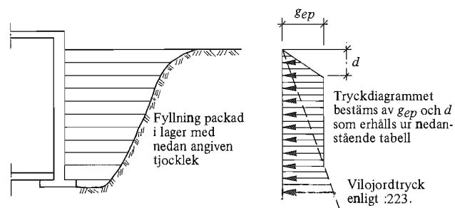
Figur 22:251. Jordtryck vid packad återfyllning av friktionsjord.
