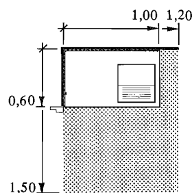
Figur 63:21 g. Tvättbänk (1,00 × 0,60 m och 1,20 × 0,60 m).
