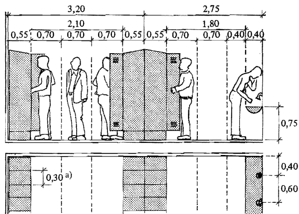
Figur 64:3 a. Exempel på minsta godtagna fria utrymmen vid klädkåp och tvättränna. - a) Vid åtskillnad mellan gång- och arbetskläder fordras större sammanlagd skåpbredd.
