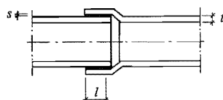
Rak överlappsfog.
