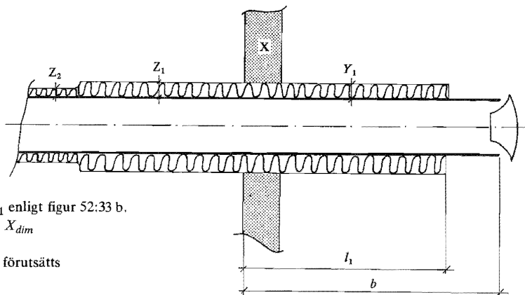
Figur 52:33 d. Godtaget genombrott till den sista brandcell som en kanal betjänar. Beteckningar enligt figur 52:33 a.
