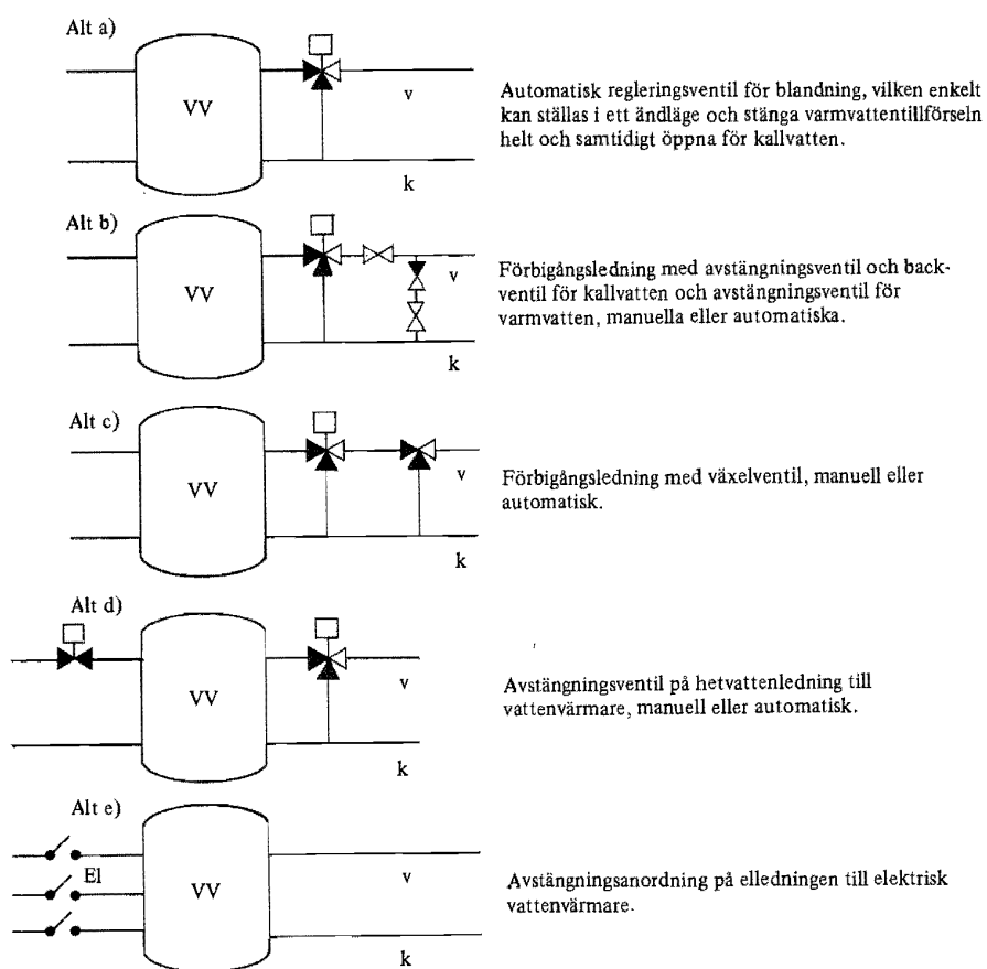
Figur 51:1662. Exempel på godtaget anordnande av kriskoppling.
