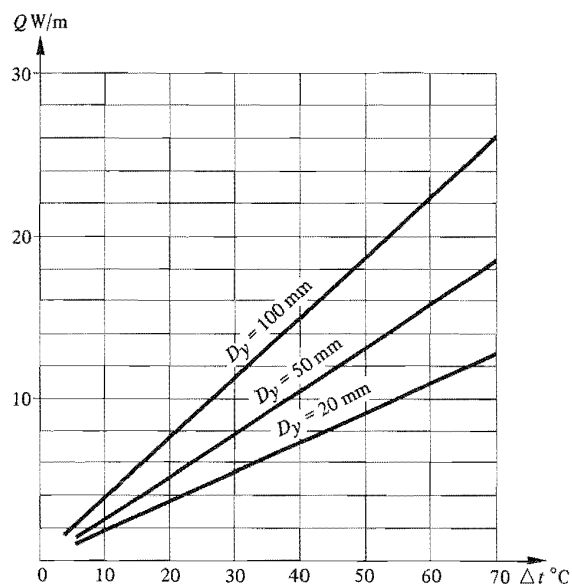
Figur 39:22. Högsta godtagna värmeavgivning Q (W/m) från friliggande isolerade rör. Beteckningar: Q värmeavgivning, W/m \Delta t temperaturskillnad, °C D_y rörets yttre diameter, mm.
