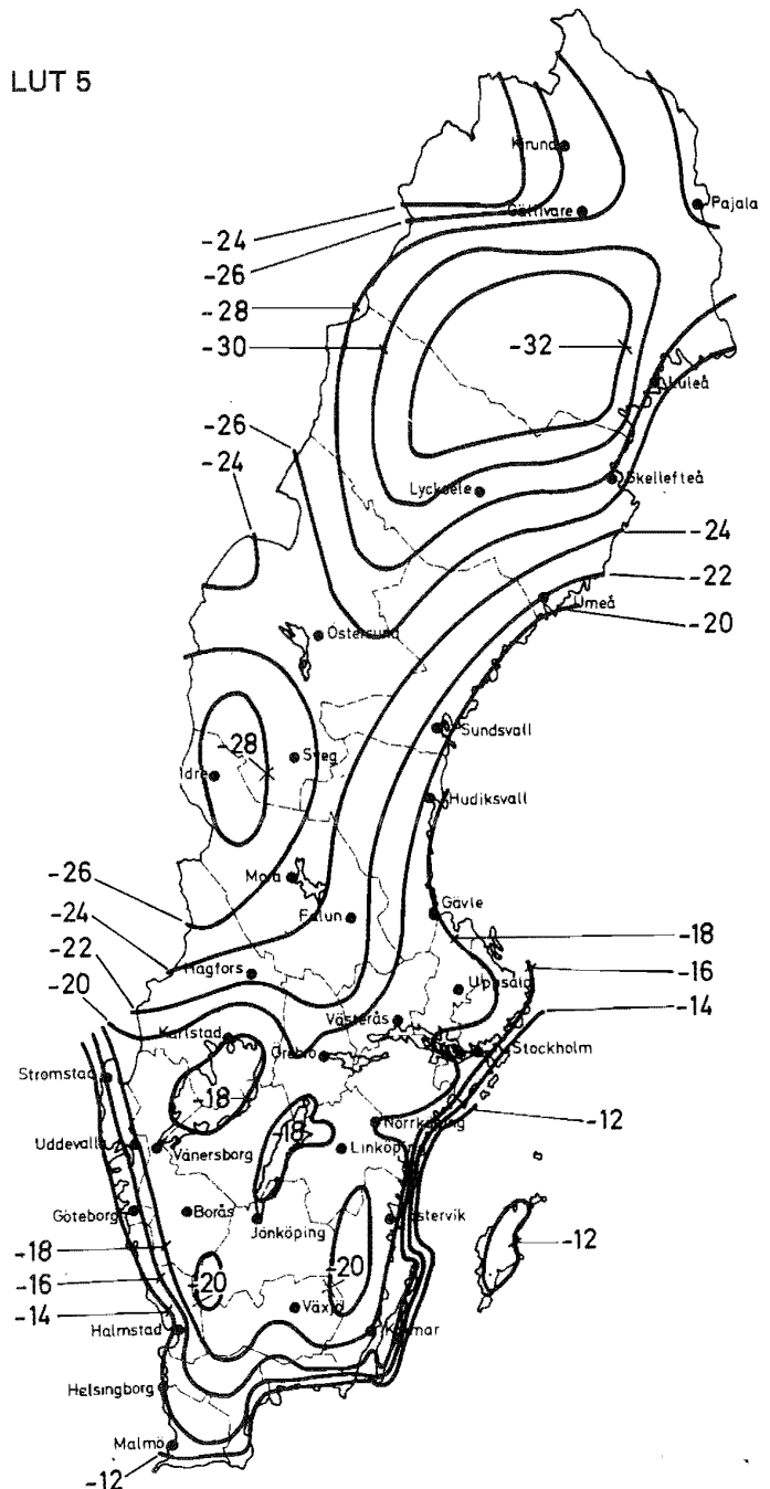
Figur 35:23 b. Isotermkarta som visar den dimensionerande lägsta utetemperaturer för hus av sten eller annan tung byggnad, LUT 5. LUT-värden enligt figuren korrigeras om ifrågakvarande byggnad ligger på en plats som bedöms vara kallare eller varmare än trakten i genomsnitt.
