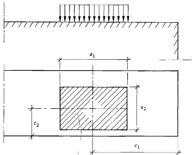
Figur 24:312. Beteckningar vid bestämning av lokalt tryck.
