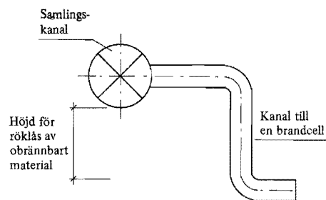
Figur 52:342. Godtagen princip för anordnande av röklås.
