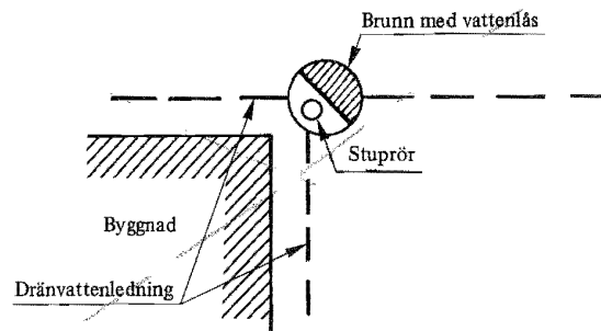
Figur 51:31 b. Exempel på godtaget sätt att ansluta dränvattenledning till dagvattenledning. Mindre installation.
