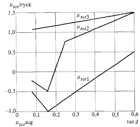
Figur 22:5344 a. Godtagna värden på formfaktorn \mu_{tot} för skärmtak med en eller flera plana ytor som lutar vinkeln \beta mot horison- talplanet. \beta antas vara minst 5^\circ .
