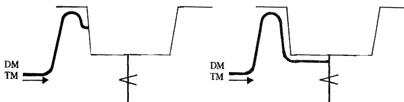
Figur 51:2432. Exempel på godtagna utföranden för anslutning av avlopp från disk- eller tvättmaskiner för hushållsbruk.
