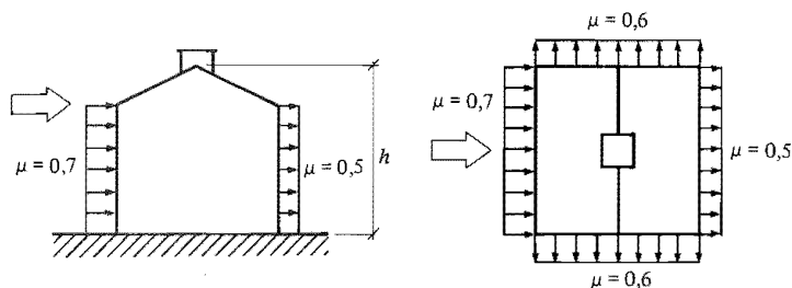
Figur 22:5331 a. Godtagna värden på formfaktorer för utvändig vindlast på ytterväggar. Höjden h används för att bestämma det exceptionella hastighetstrycket enligt figur 22:52.
