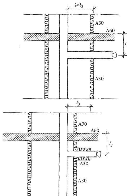
Figur 52:331 a. Godtaget utförande av en isolerad kanal i ett stängt schakt. Beteckningar enligt figur 52:33 a. Villkor enligt figurerna 52:33 b-c.
