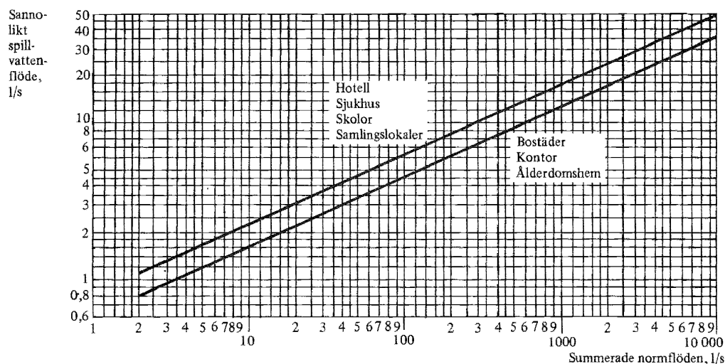
Figur 51:251. Sannolikt spillvattenflöde som funktion av summerade normflöden. I diagrammet har hänsyn tagits till att samtliga till en ledning anslutna avloppsenheter inte används samtidigt. Vid summerade normflöden mindre än 10 l/s kontrolleras att det sannolika flödet inte är mindre än det största enskilda normflödet.
