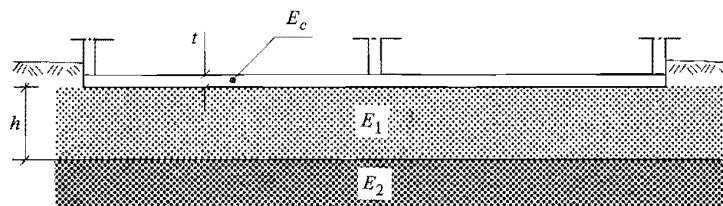
Figur 23:262 c. Beräkning av ekvivalent elasticitetsmodul för två jordlager med elasticitetsmodulerna E_1 och E_2 .
