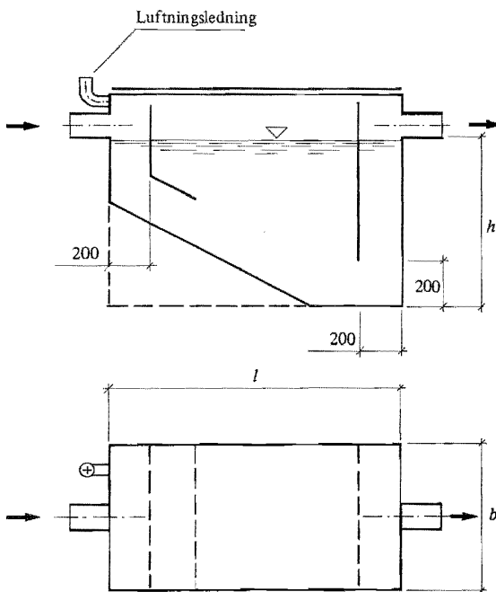
Figur 51:223 b. Godtagna dimensioner för oljeavskiljare och fettavskiljare (mm). Principskiss. Jfr tabell 51:223 d.
