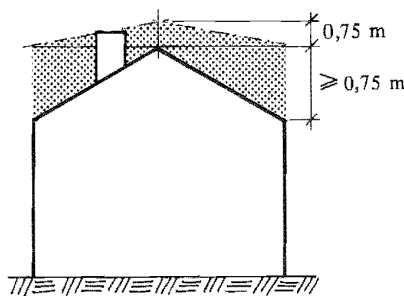
Figur 44:121 b. Godtagen höjd över yttertak för rökkanal till en öppen spis eller en kamin i småhus, som huvudsakligen värms upp med annan anordning.
