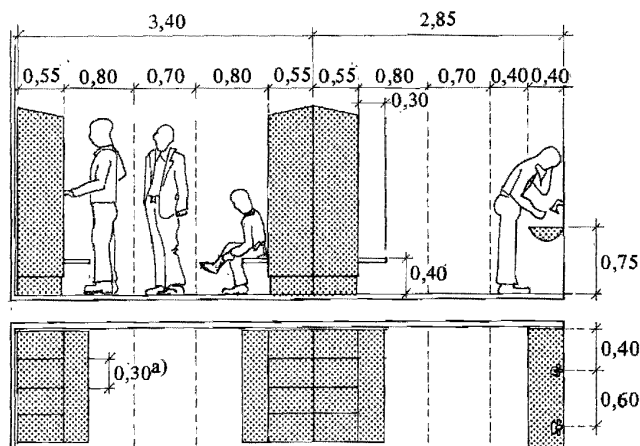
Figur 64:3 b. Exempel på minsta godtagna fria utrymmen vid klädkåp med sittbänk och tvättränna. - a) Vid åtskillnad mellan gång- och arbetskläder fordras större sammanlagd skåpbredd.
