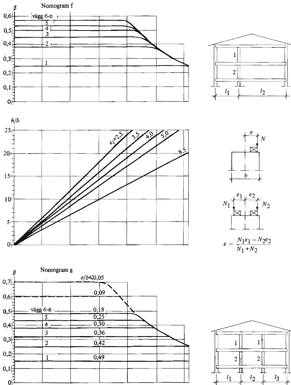
Figur 24:422 f-g. Godtagna reduktionsfaktorer för väggar med från båda sidor anslutande bjälklag (innerväggar) eller då e/b är känt. Nomogram f gäller vid enkelspända bjälklag i byggnader med två fack när l_1/l_2 \leq 0,8 och l_2 \leq 5,0 m. Nomogram g gäller vid enkelspända bjälklag i byggnader med tre eller flera fack med spännvidden högst 5 m samt där e bestäms enligt figuren.
