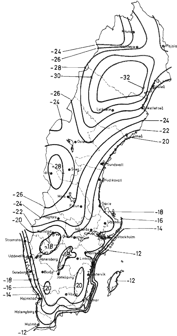
Figur 22:721. Godtagna dygnsmedelvärden för låga temperaturer.
