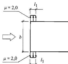
Figur 22:5331 a. Godtagna värden på formfaktorer för utvändig vindlast på ytterväggar. Höjden h används för att bestämma det exceptionella hastighetstrycket enligt figur 22:52.
