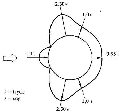
Figur 22:5341 c. Godtagen fördelning av vindlastintensiteten kring stänger med cirkulärt tvärsnitt, när \mu_{tot} = 0,7 som svarar mot \frac{u}{d} = 4 \cdot 10^{-4}
