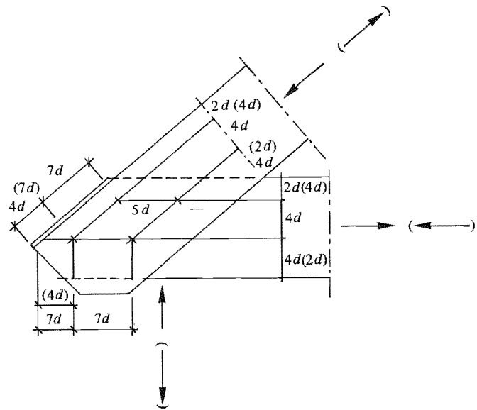
Figur 27:54. Förutsatta minimiavstånd mellan skruvar och från skruv till virkeskant i skruvförband utan mellanlägsbrickor. Värden inom parentes gäller för inom parentes angiven kraftpåverkan. ( d är skruvdiameter.)
