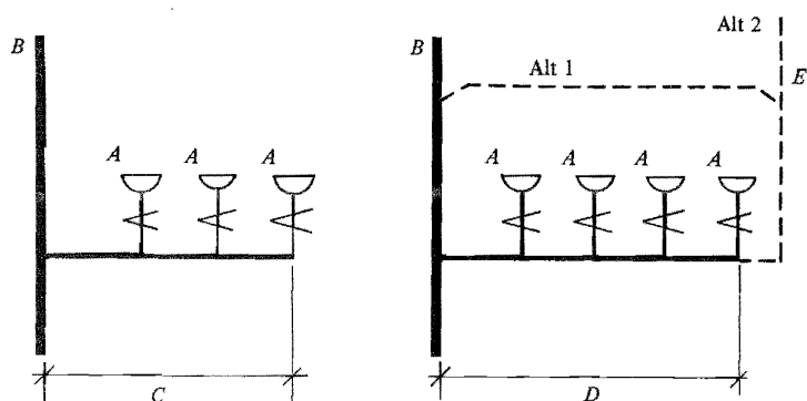
Figur 51:261 b. Exempel på luftning av ledning
