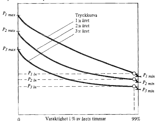
Figur 51:13. Definition av lägsta normala vattentryck.
