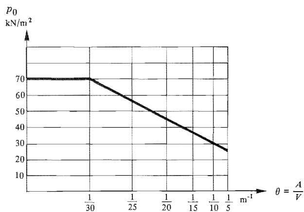
Figur 22:84. Antagna invändiga övertryck i en enda sluten lokal som funktion av faktorn \theta .
