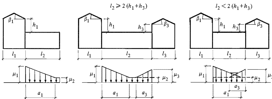
Figur 22:43 c. Godtagna formfaktorer för snölast vid skärm. Beträffande förutsättningar se faktaruta ovan.
