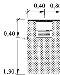
Figur 63:21 f. Tvättlåda (0,40 × 0,40 m).
