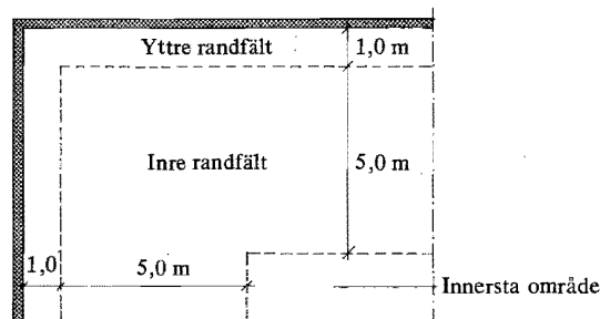
Figur 33:247. Fältindelning av golv på mark.
