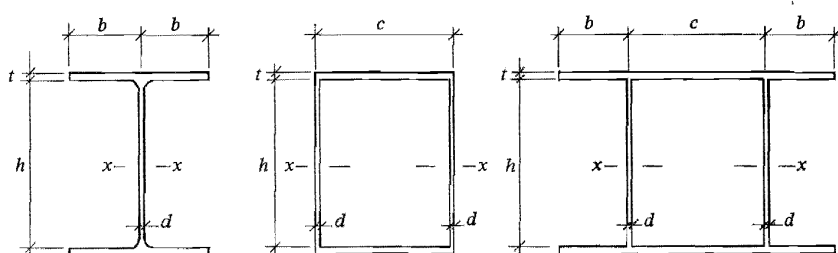
Figur 28:21. Beteckningar för tvärsnittsmått.
