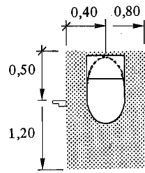
Figur 63:21 c. Wc-stol eller bidé (0,40 × 0,70 m).
