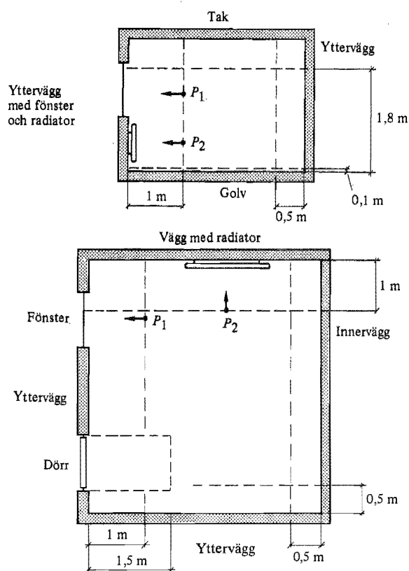
Figur 35:21. Exempel som visar kontrollzonens storlek och placering av punkterna P_1 och P_2 enligt 35:21.
