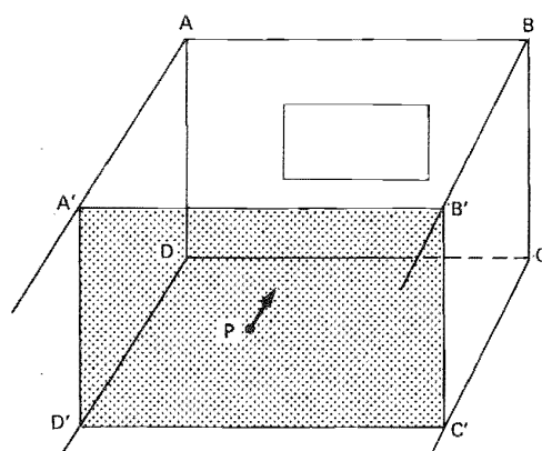
Figur 35:22 a Förklaring av begreppet medelstrålningstemperatur \bar{\vartheta}_y . Utgående från en punkt P läggs ett plan med valfri riktning. Varje ytans bidrag till \bar{\vartheta}_y ges av ytans temperatur beräknad enligt formel 35:23 multiplicerad med ytans vinkelkoefficient \varphi med avseende på punkten P och det valda planet. För beräkning av \varphi se figurer 35:22 b och c.
