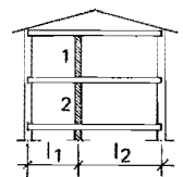
Figur 24:422 d - e Faktor vid väggar med från båda sidor anslutande bjälklag (innerväggar).
