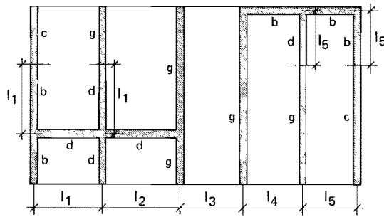
Figur 24:422 a Väggarpartier b, c, d och g för vilka nomogrammen i figurer 24:422 b – g gäller.
