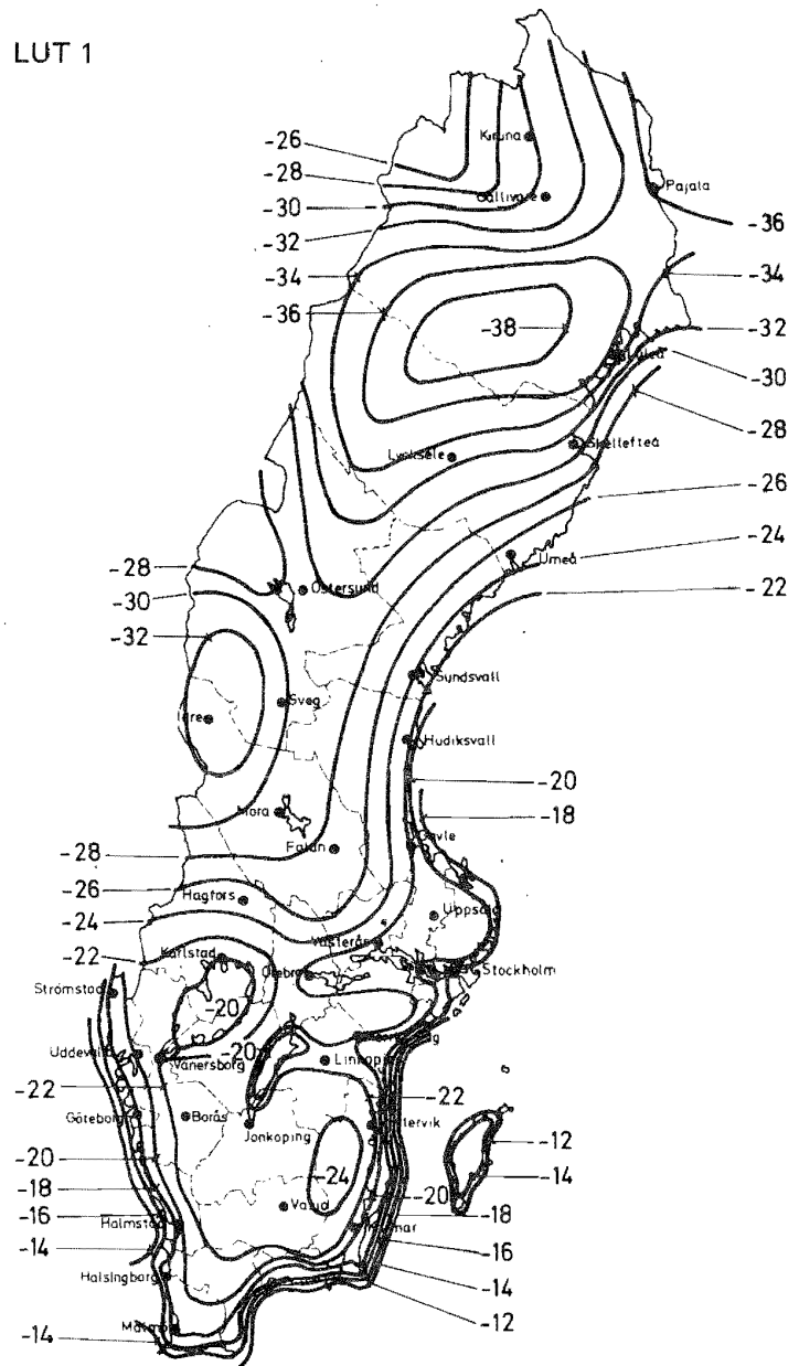
Figur 35:23 a Isotermkarta visande dimensionerande lägsta utetemperatur för hus av trä eller annan lätt byggnad, LUT 1. LUT-värden enligt figuren korrigeras om ifrågasatt byggnad ligger på en plats som bedöms vara kallare eller varmare än trakten i genomsnitt.
