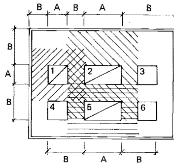
Figur 44:324 b Kanalerna 1 och 2 är rökanaler från värmepannor eller liknande eldstäder. Kanalerna 3, 4 och 6 är ventilationskanaler. Kanal 5 är rökanal från öppen spis. Erforderliga kanalväggar är streckmarkerade. Mitt för rökanal (områden betecknade A) får brännbart material inte anslutas. Mot områden betecknade B får väggkonstruktion utförd enligt alternativ I och II i figur 44:324 a anslutas. Mot övriga områden får brännbart material anslutas.
