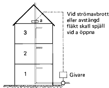
Figur 52:342 a Anordnande av spjäll då frånluftsfläkt placeras under eller i samma plan som anslutna brandceller.
