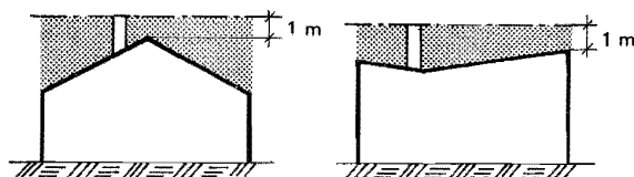
Figur 44:121 Rökanals höjd över tak om ansluten eldstad har en tillförd värmeeffekt av högst 60 kW.
