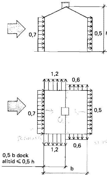
Figur 21:6331 Formfaktorer för utvärdig vindlast på ytterväggar och höjd h för bestämning av hastighetstryck enligt :62.
