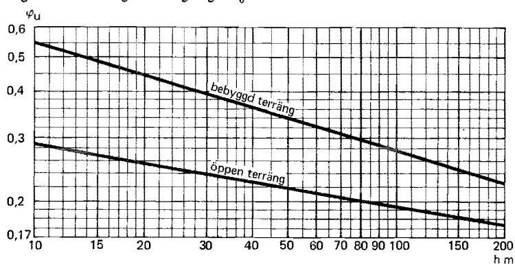
Figur 21:642 b Vindlastens råhetsfaktor som funktion av konstruktionens höjd h över marken och terrängens struktur.
