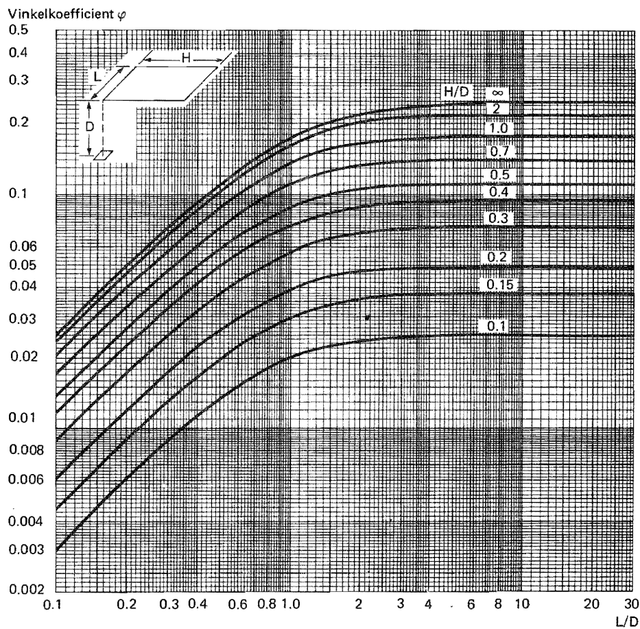
Figur 35:22 b Vinkelkoefficienten \varphi vid strålning mellan en liten yta och en med denna parallell större yta.
