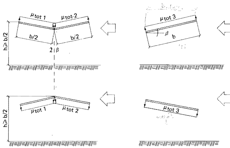
Figur 21:6344 Formfaktor \mu_{tot} för skärmtak som lutar vinkeln \beta mot horisontalplanet. \beta antas vara > 5^\circ .
