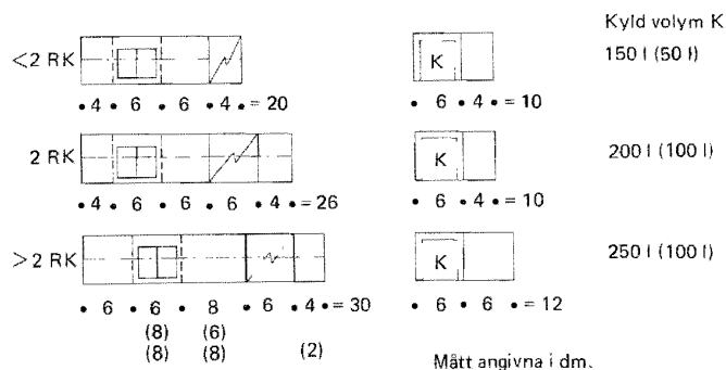
Figur 71 Omb: 214 Köksutrustningsmängd för olika lägenhetsstorlekar. Delmått anges i dm (alternativa kombinationer inom parentes).
