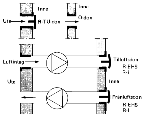
Figur 36:42 Förklaring av benämningar på don.
