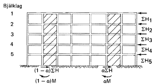
Figur 22:44 b Plan och längdsnitt genom en byggnadsstomme för flervåningsbyggnad. Figuren visar i byggnadens längdled verkande horisontalkrafter H. Varje pil petecknar en H-kraft där ej annat anges. Lutande streckmarkering betecknar i horisontalled stabiliserande konstruktion. \Sigma H_v betecknar summan av H-kraften under bjälklag v.
