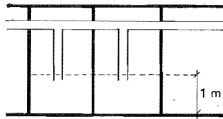
Figur 52:341 a Till- eller frånluftsdon placeras högst 1 m ovan golv.
