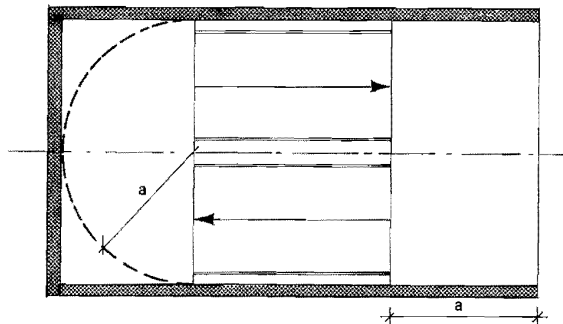
Figur 62:23 Trapplans bredd
