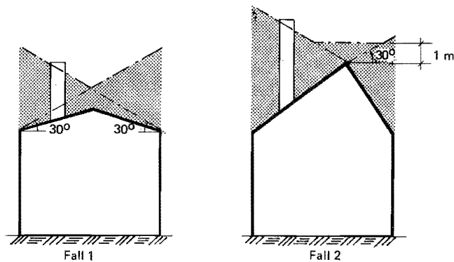
Figur 44:1222 Beräkning av höjd för röckkanal till panncentral med tillförd värmeeffekt 0,06 < P \leq 50 MW, tunnolja.
