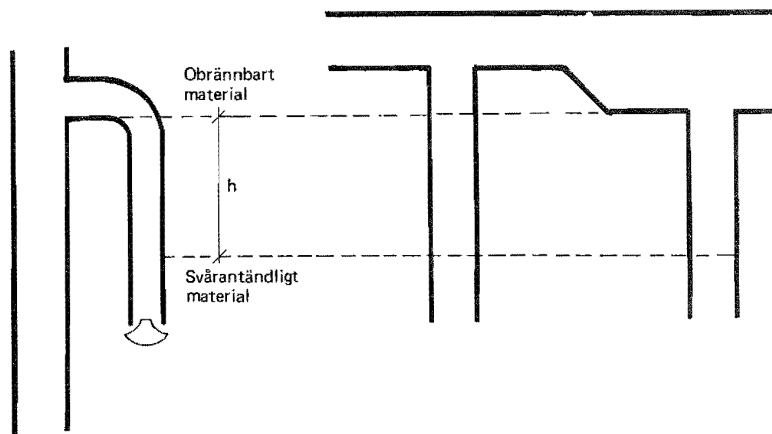
Figur 52:342 b.Princip för anordnande av röklås.
