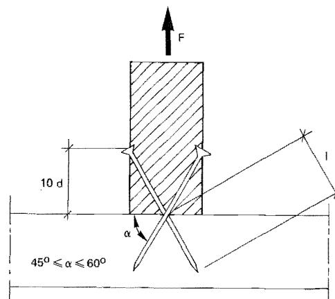
Figur 27:2223 b Skråspikning.
