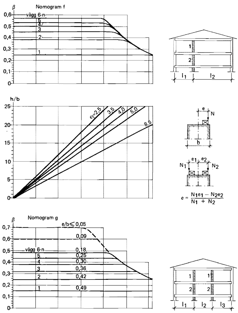
Figur 24:422 f-g Faktor vid väggar med från båda sidor anslutande bjälklag (innerväggar) eller då e/b är känt.
