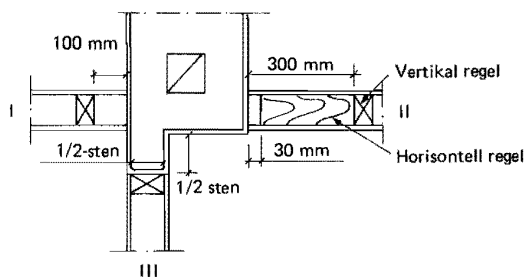
Figur 44:324 a Väggsanslutningar till rökkanalens omslutningsvägg. Vid alternativ I (vägg med vertikala regler) skall regel befinna sig minst 100 mm från rökkanalens omslutningsvägg. Vid alternativ II (vägg med horisontella regler) skall ändtytor på regler befinna sig minst 30 mm från omslutningsväggen och eventuell vertikal regel e d minst 300 mm från väggen. Vid alternativ III får såväl väggpanel som träregel anslutas direkt mot murklack.
