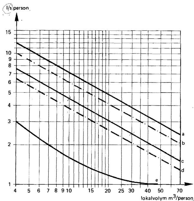
Figur 36:22 Godtagna uteluftsflöden.
