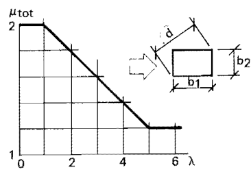
Figur 21:6341 a Formfaktorer för rektangulära stänger med 1 > 5 d och \lambda = b_1/b_2 .
