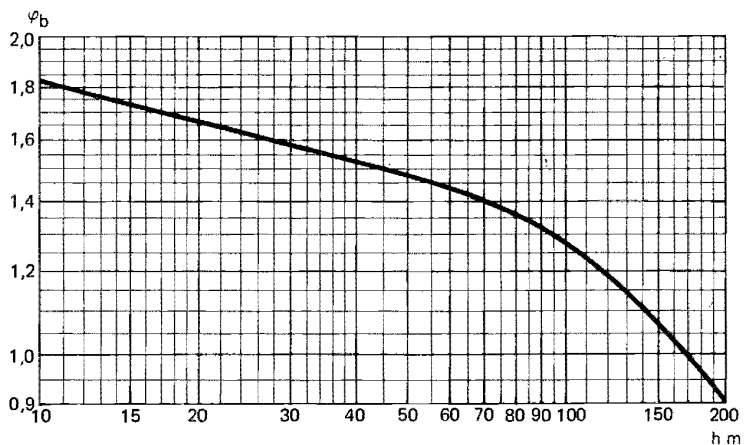
Figur 21:642 c Vindlastens stimulans från bakgrundsturbulensen som funktion av konstruktionens höjd h över marken.
