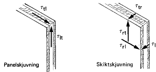
Figur 27:213 a Skjuvpåverkan vid plywood: Panelskjuvning Skiktssjuvning
