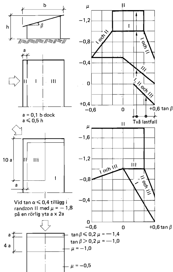
Figur 21:6332 b Formfaktorer för utvändigt vindlast på pulpettak och höjd h för bestämning av hastighetstryck enligt :62. Undertryck betecknas negativt, övertryck positivt.
