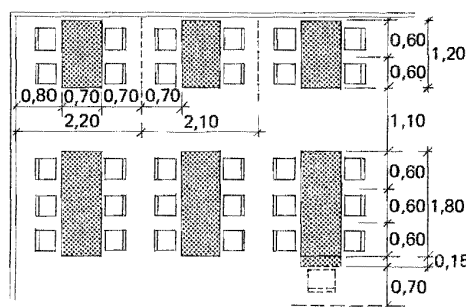
Figur 64:2 Minsta godtagbara mått för bord, gångar m m i matrum. Mått i meter.
