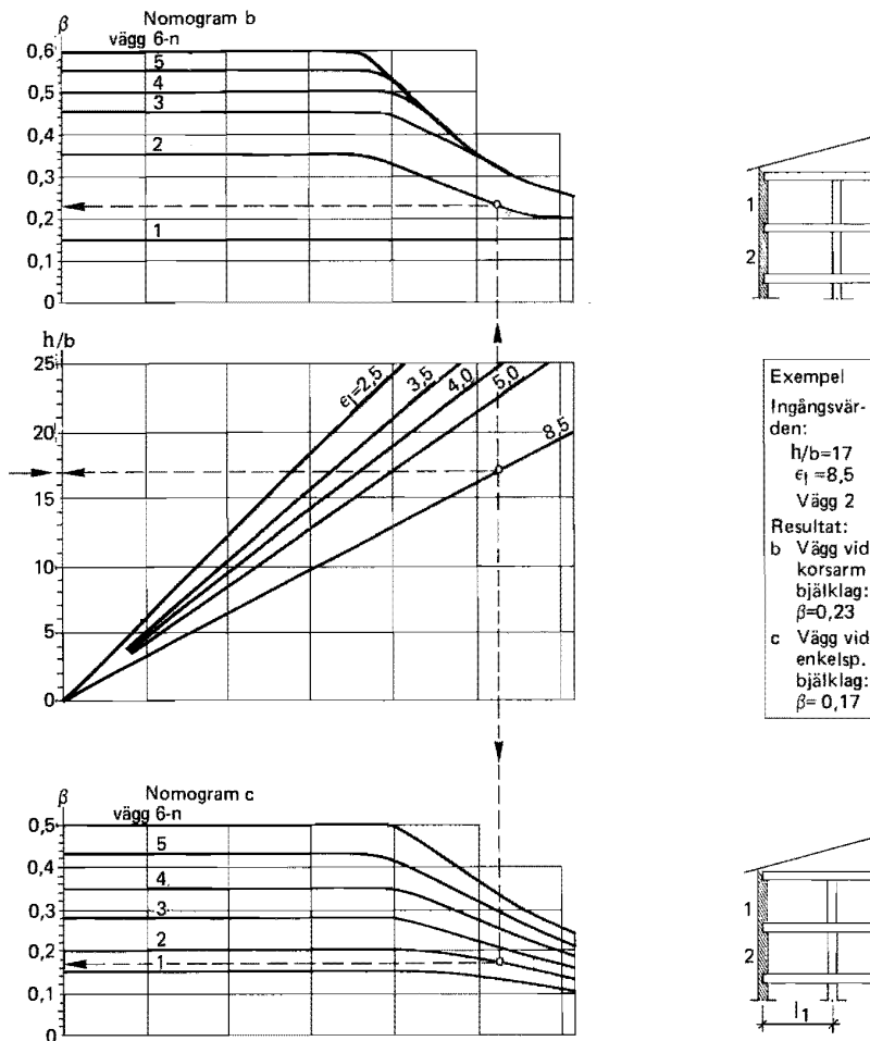
Figur 24:422 b – c Faktor vid väggar med från en sida anslutande bjälklag (ytterväggar och liknande). Nomogram b gäller vid korsarmerade bjälklag med minsta spännvidden max 5,0 m. Nomogram c gäller vid enkelspända bjälklag! \leq 5,0 m.
