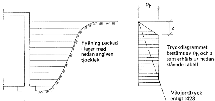
Figur 21:451 Jordtryck vid packad återfyllning av friktionsjord.
