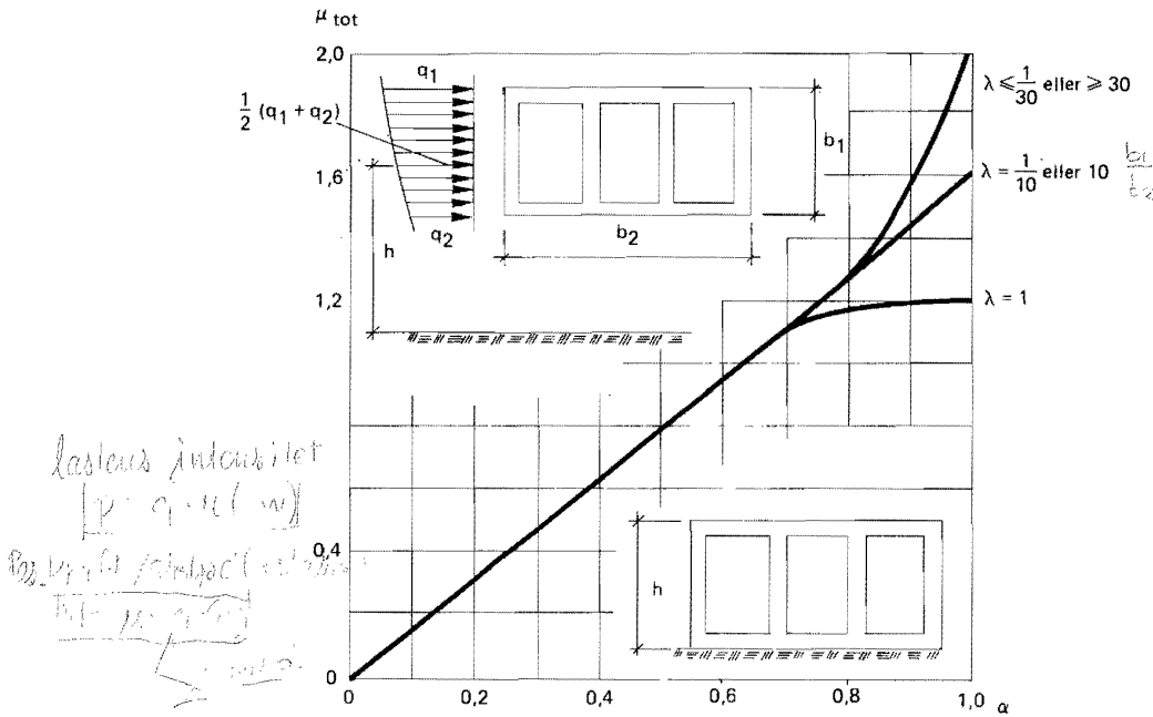
Figur 21:6342 a Formfaktor för en skärm med kantiga stänger. \alpha = A_p/A där A_p är nettoarean av anblåsta stänger i skärmen och A är skärmens bruttoarea. \lambda = b_1/b_2 För skärmar med markkontakt gäller figuren endast för b_1/b_2 = h/b_2 < 2 .
