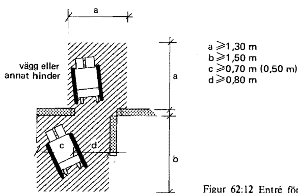
Figur 62:12 Entré för passage med rullstol
