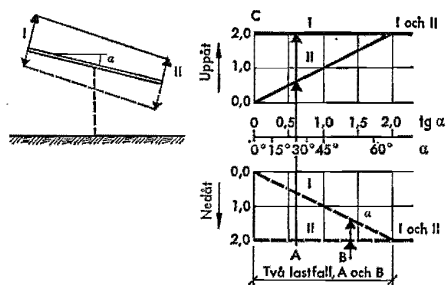
Fig 21:6334 Formfaktor C för fristående pulpettak
