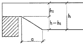
Fig 27:263 Inskärning vid upplag
