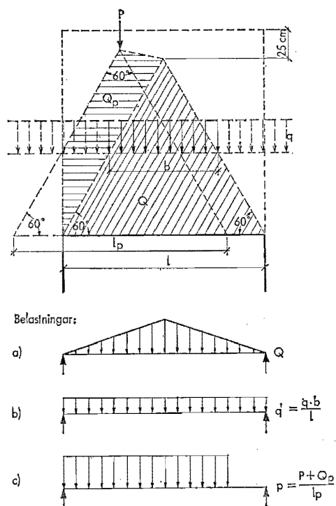
Fig 24:4411 Laster för beräkning av bärande konstruktion över öppning.
