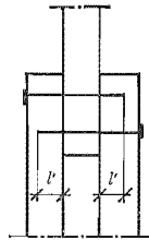
Fig 27:321b Tvåskärigt förband med spikar i fogen slagna från båda sidor.
