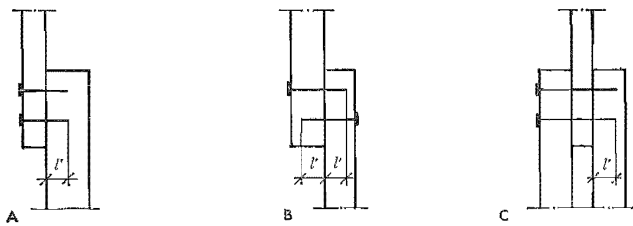
Fig 27:321a Enskärigt förband (A och B) och tvåskärigt förband med spikar i fogen slagna från en sida (C).
