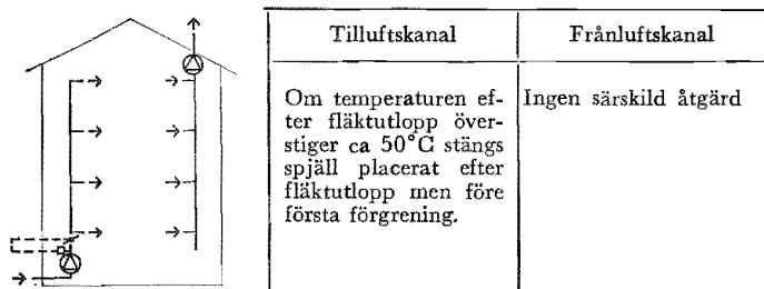
Fig 36:15212 e Godtagbara åtgärder vid kanalers förening: FT-ventilation, tilluftsläkt ej vindsplacerad, frånluftsläkt vindsplacerad.
