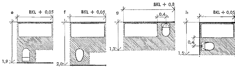
Fig 63:25 e-h Badkar och wc-stol eller bidé.
