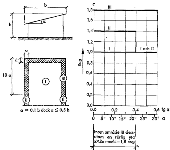
Fig 21:63234 Formfaktor c för pulpettak
