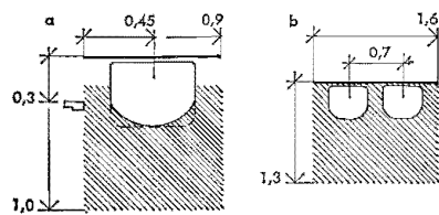
Fig 63:21a Tvättställ 0,60×0,45 m. Fig b Två tvättställ.
