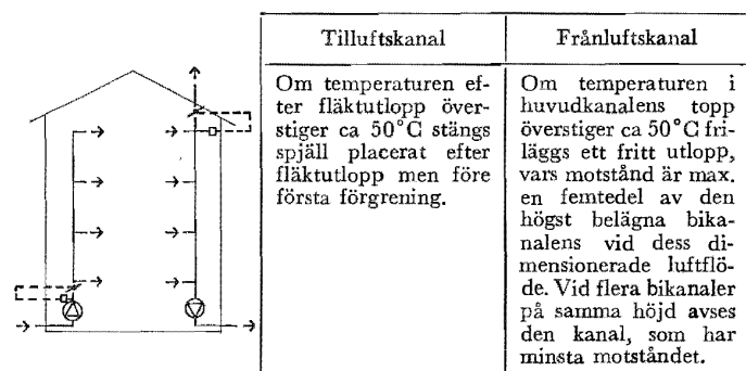
Fig 36:15212 f Godtagbara åtgärder vid kanalers förening: FT-ventilation, fläktar ej vindsplacerade.
