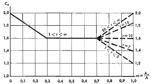
Fig 21:6363 Formfaktor C_a vid enstaka skärm utan markkontakt
