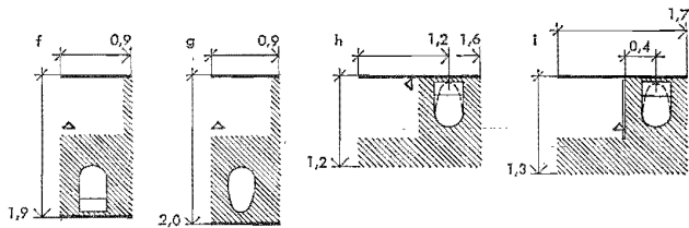
Fig 63:26 f-i Duschplats och wc-stol eller bidé.
