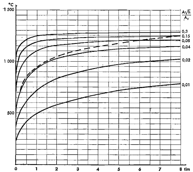
Fig 37:123 Samband mellan brandcellstemperatur \vartheta_s och brandtid t för varierande öppningsfaktor A\sqrt{h}/A_1
