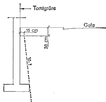
Fig 23 :222 Mått för grundkonstruktions utformning i gräns mot gata
