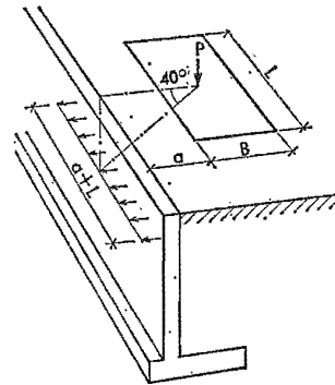
Fig 21:432 Angreppslinje och utbredning för jordtryck av koncentrerad last
