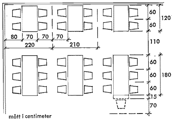
Fig 64:41 Lämpliga mått för bord, gångar m m i matrum.
