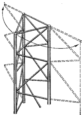
Fig 21:6365 Vindyta vid fackverksmast av runda stänger
