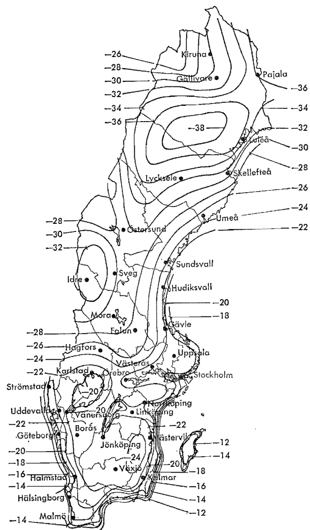
Fig 35:3a Isotermkarta med dimensionerande utetemperatur för värmeanläggning, DUT 1
