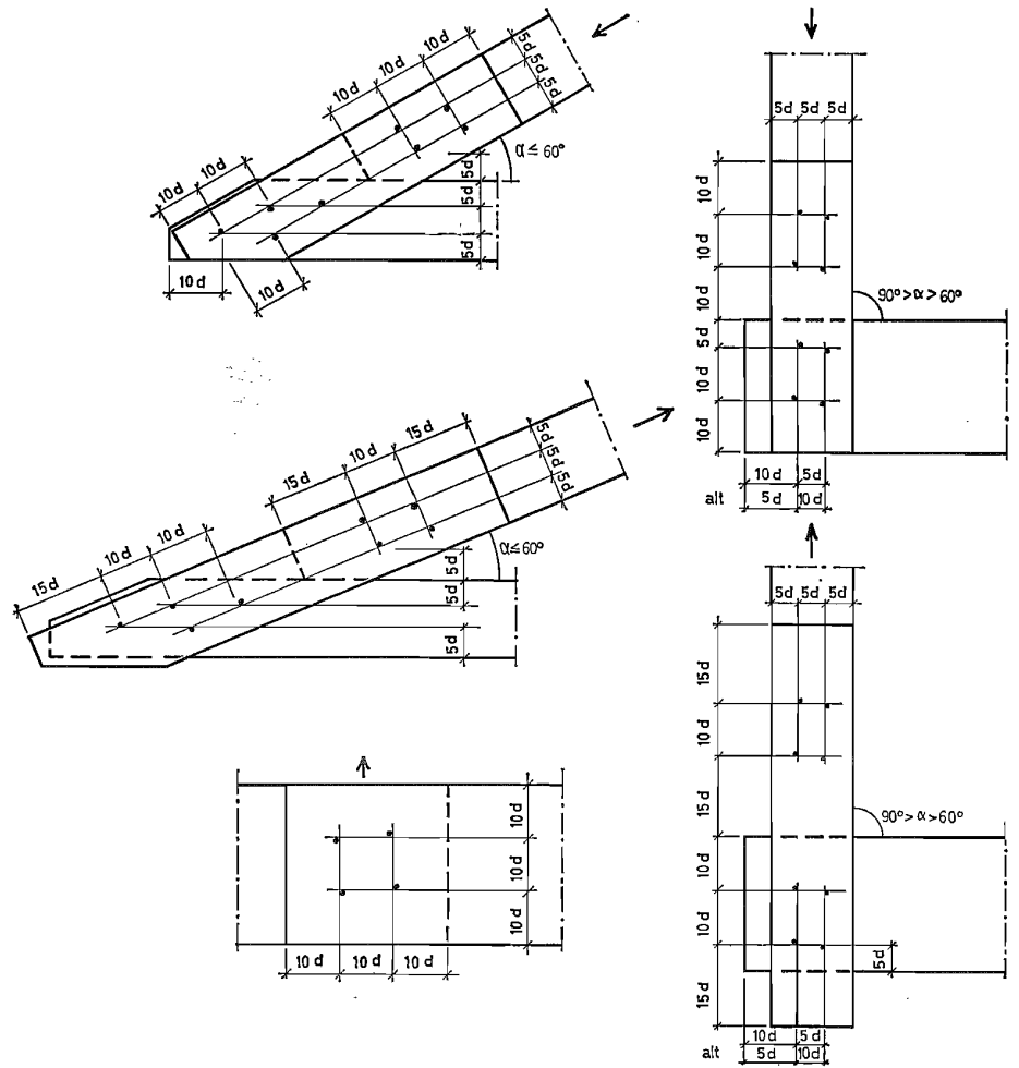
Fig 27:321c Minsta spikavstånd vid olika typer av anslutningar
