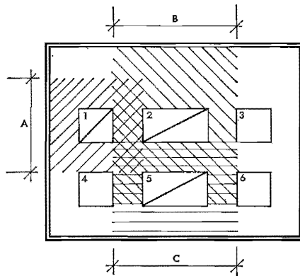
Fig 44:324 Kanalerna 1 och 2 är rökkanaer från värmeplattor eller liknande eldstäder. Kanalerna 3, 4 och 6 är ventilationskanaler. Kanal 5 är rökkana från öppen spis. Områdena A, B och C är de delar av skorstenens tvärsnittsyta som skall anses utgöra omslutningsväggar till kanalerna 1, 2 resp 5.
