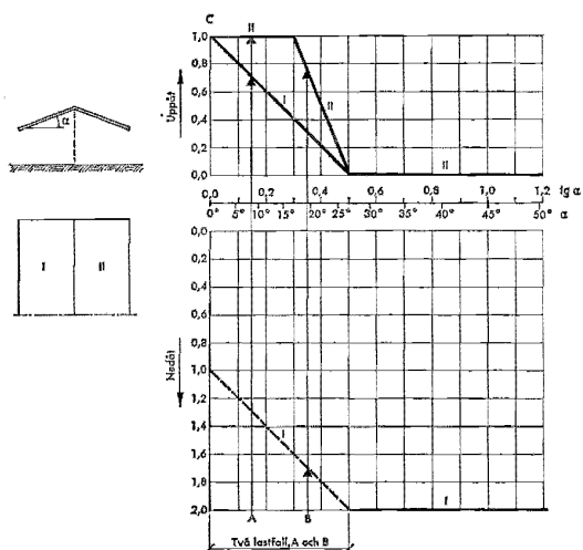
Fig 21:6332 Formfaktor C för fristående sadeltak
