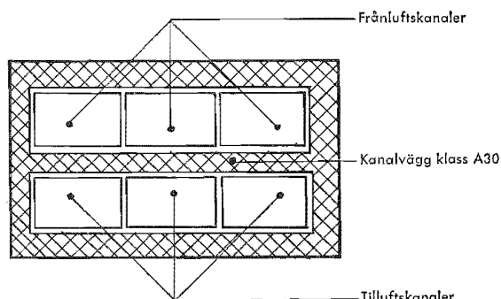
Fig 36:15441 Exempel på kanalers avskiljande i schakt
