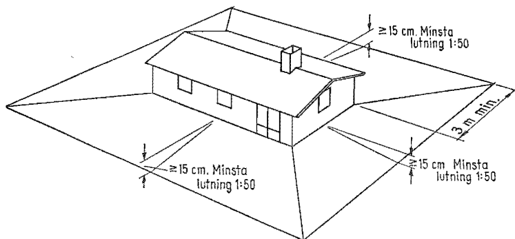
Fig 32:2211. Exempel på lämplig lutning på markytan kring byggnader med golv direkt på mark enligt Byggeforskningens småskrift nr 22.
