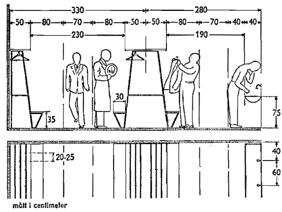
Fig 64:221 b Erforderliga fria utrymmen vid klädställning och tvättränna.
