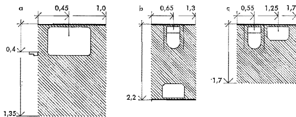
Fig 63:41 a Tvättställ 0,70 x 0,50 m. Fig b, c Tvättställ och wc-stol.
