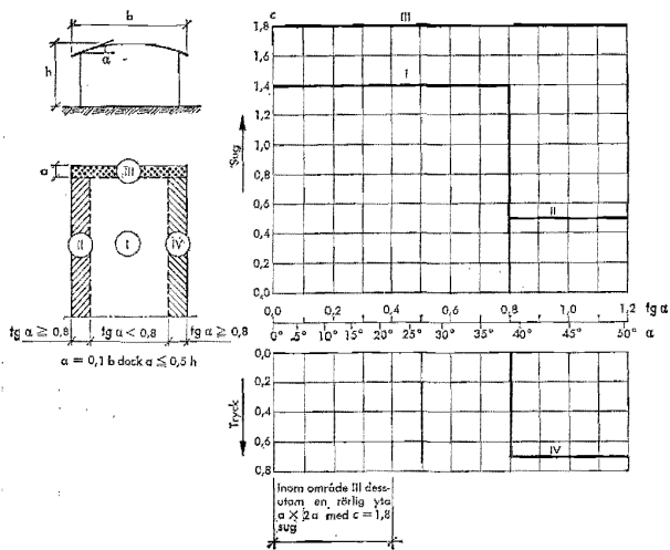
Fig 21:63235 Formfaktor c för bågtag med pilhöjdsförhållandet minst 1:8.
