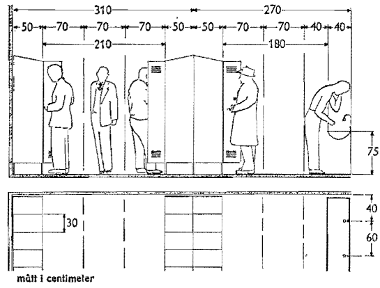
Fig 64:221 a Erforderliga fria utrymmen vid klädskåp och tvättränna.
