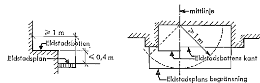
Fig 45:25 Eldstadsplan framför öppen spis, vertikalsektion och plan.
