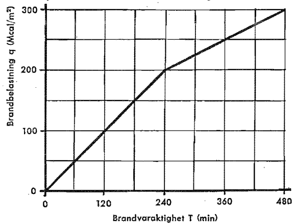
Fig 37:122 Samband mellan brandbelastning q och brandvaraktighet T
