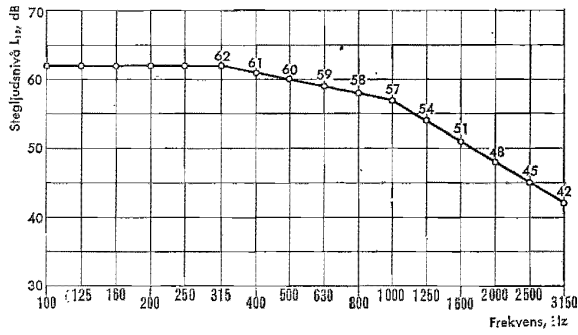
Fig 34:024 a Referenskurva för stegljudsnivå L_{10} .
