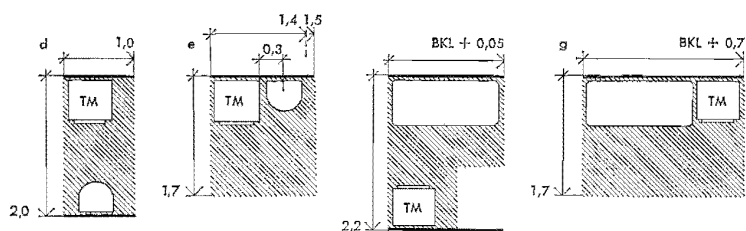
Fig 63:33 d, e Tvättmaskin och tvättställ. Fig f, g Tvättmaskin och badkar.
