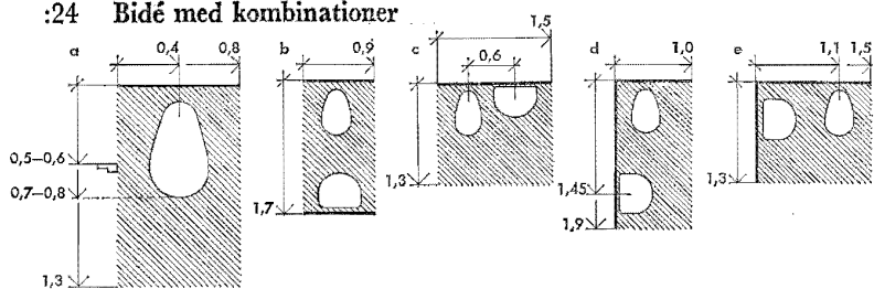
Fig 63:24 a Bidé 0,40×0,65 m. Avståndet mellan framkant och vägg bakom bidén görs minst 0,70 m (helst 0,80 m). Fig b-e Bidé och tvättställ.
