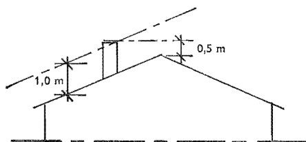
Fig 36:1431 Ventilationskorstens höjd över tak
