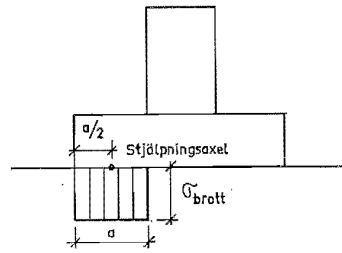
Fig 22:331 Bestämning av stjälpningsaxelns läge vid grundläggning på jord.
