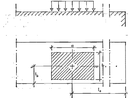
Fig 24:4434 Lokalt tryck
