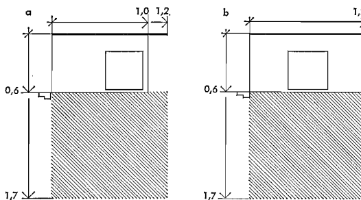
Fig 63:32 a Tvättbänk 1,00 × 0,60 m. Avståndet mellan tvätthons mitt och vägg eller högskåp görs minst 0,40 m.
