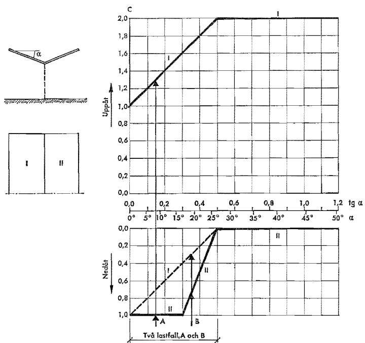
Fig 21:6333 Formfaktor C för fristående omvända sadeltak
