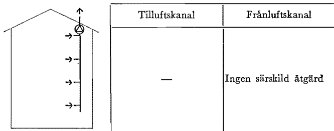
Fig 36:15212 a Kanalers förening: F-ventilation, fläkt vinds-placerad.
