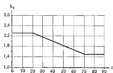
Fig 27:2732 Faktor k_f vid olika slankhetstal
