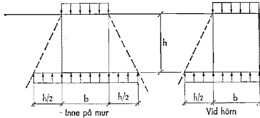
Fig 24:441 Tryckutbredning under upplag.
