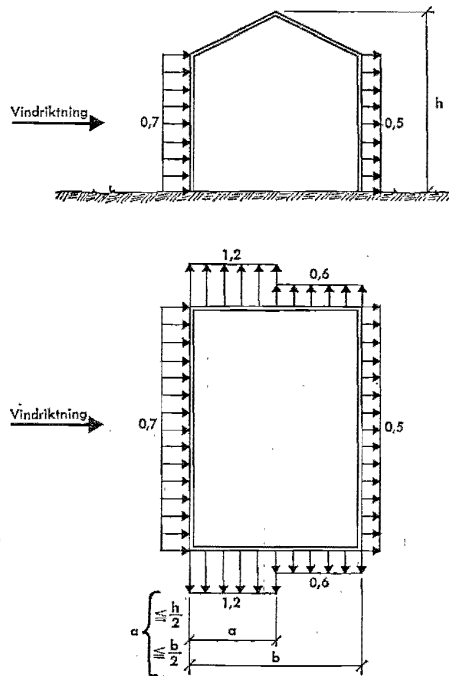
Fig 21:63231 Formfaktor c för yttervägg
