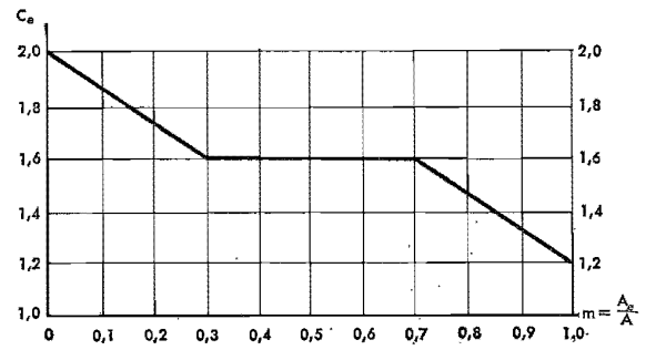
Fig 21:6362 Formfaktor C_a vid enstaka skärm med markkontakt
