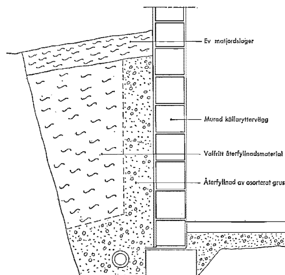
Fig 32:2222 Exempel på återfyllnad utanför murad källarytervägg.
