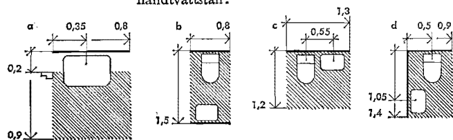
Fig 63:23a Handtvättställ 0,50×0,35 m. Fig b-d Handtvättställ och wc-stol.
