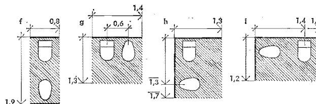
Fig 63:24 f-i Bidé och wc-stol.
