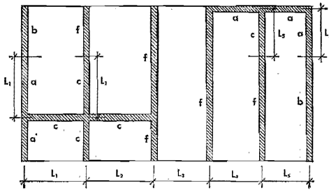
Fig 24:44322 g) \beta -nomogram vid olika väggpartier
