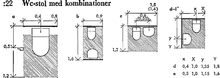
Fig 63:22 a Wc-stol 0,40×0,70 m.
