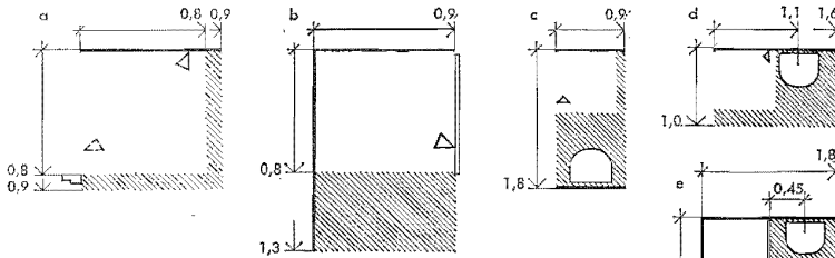
Fig 63:26 a Duschplats 0,80 x 0,80 m. På tre sidor fast avskärmad duschplats görs 0,90 x 0,80 m, slutet duschutrymme 0,90 x 0,90 m. Fig b Duschplats med fast skärm. Fig c-e Duschplats och tvättställ.
