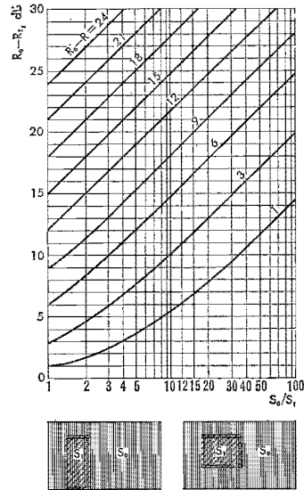
Fig 34:423 Diagram för beräkning av resulterande ljudisolering. R_o = väggens reduktionstal, R_i = fönstrets (dörrens) reduktionstal, S_o = väggens yta inkl fönster (dörr), S_i = fönstrets (dörrens) yta. Exempel: I en vägg med R_o = 50 dB insätts ett fönster med R_i = 25 dB ( R_o - R_i = 25 dB). Fönsterytan är 20 % av väggytan inkl fönster ( S_o/S_i = 5 ). Enligt diagrammet minskar väggens isolering ( R_o - R ) med 18 dB, dvs från 50 till 32 dB.
