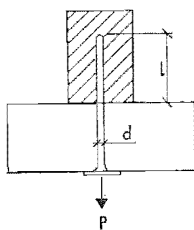
Fig 27:323 Axiell last på spik
