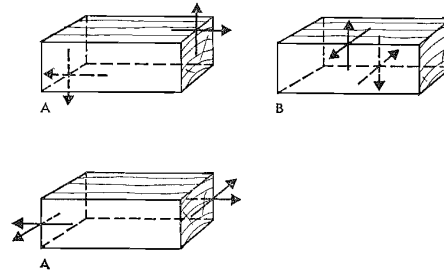
Fig 27:25 Skjuvning vid konstruktionsvirke
