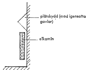
Fig 13:2231 Exempel på skydd över uppvärmningsanordning
