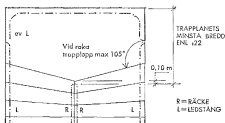
Fig 62:13 Trappplan vid trappa med kilformiga steg.
