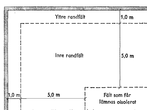
Fig 33:251. Fältindelning av golv direkt på mark
