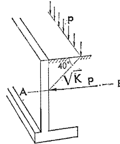
Fig 21:431 Angreppslinje för jordtryck av linjelast
