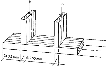
Fig. 27:222 Minsta avstånd vid syll- och stämpeltryck
