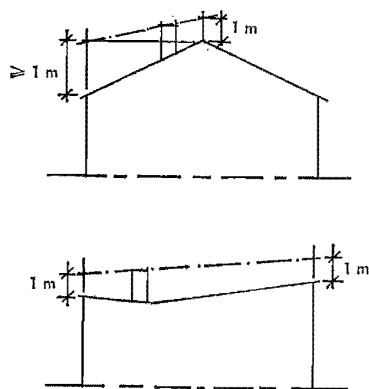
Fig 44:1211 Rökkanals höjd över tak om ansluten eldstad har en tillförd värmeeffekt av högst 50 Mcal/h.
