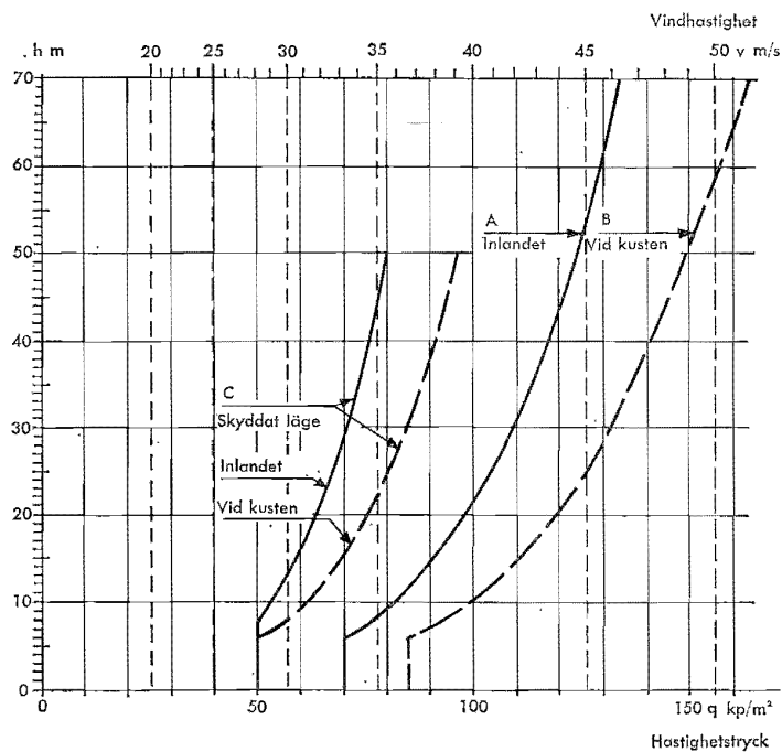
Fig 21:621 Dimensionerande vindhastighet och hastighetstryck
