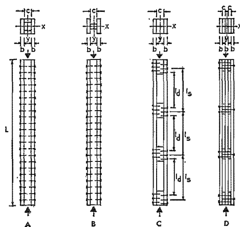
Fig 27:2731 Sammansatta stänger
