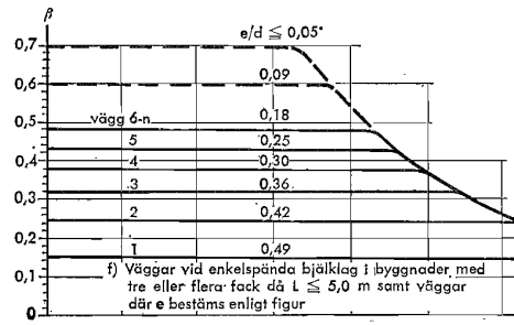
Fig 24:44322 e och f Faktor \beta vid väggar med från båda sidor anslutande bjälklag (innerväggar) eller då e/d är känt.
