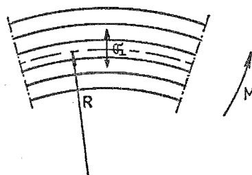
Fig 27:233 Dragpåkänning i tvärled vid krökt element.
